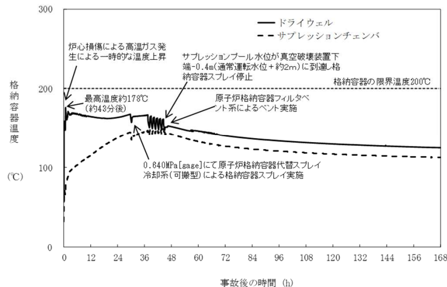
図2-2 格納容器温度の推移
