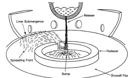
BWR Mark-I型格納容器の溶融炉心の流出イメージ [2]
