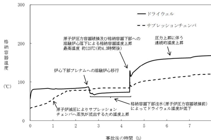
図3-4 格納容器温度の推移
