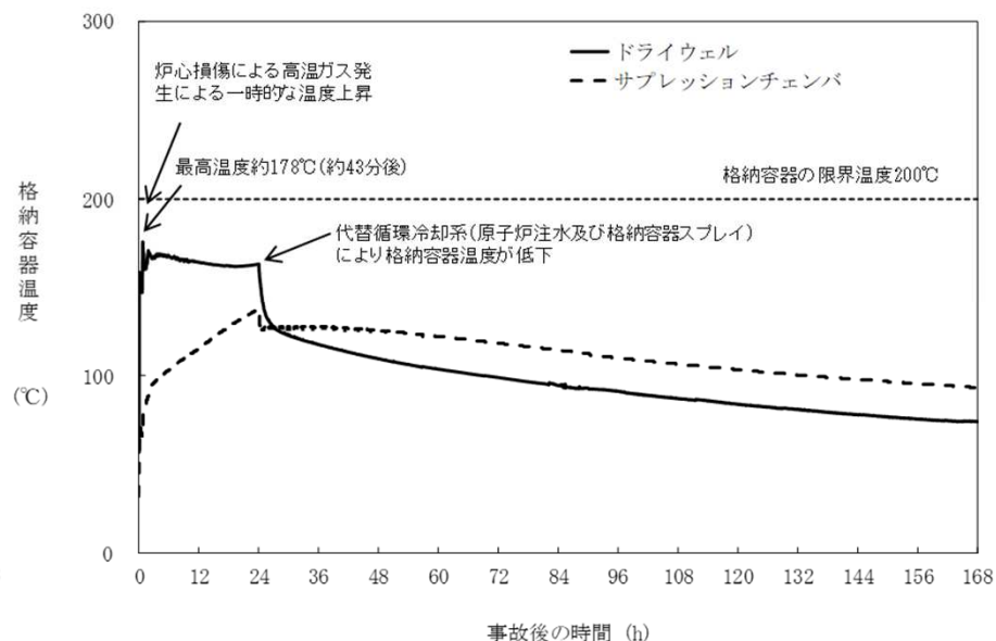
図1-2 格納容器温度の推移
