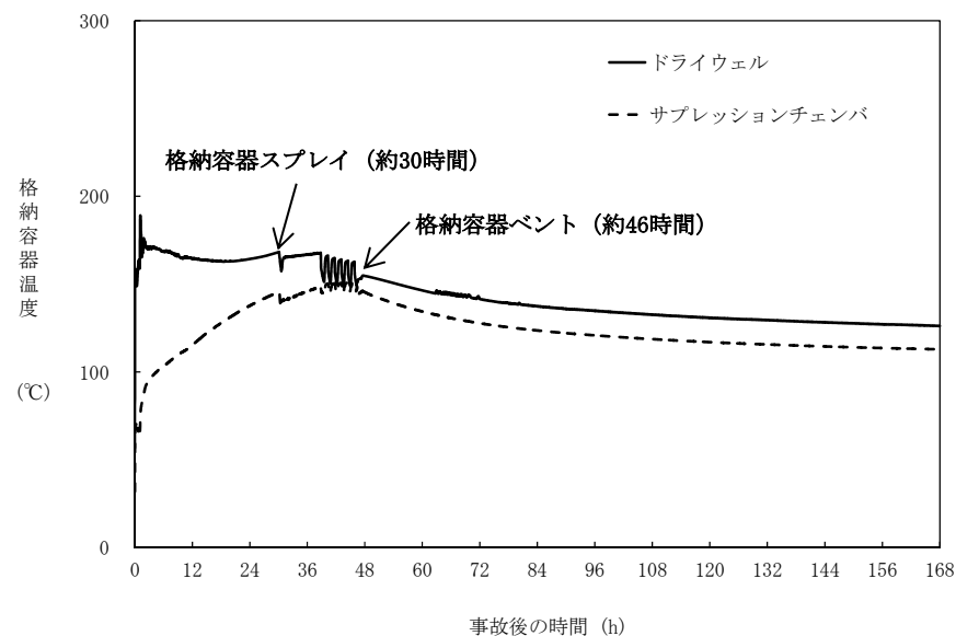
図2-4 操作25分遅れのケースにおける格納容器温度の推移
