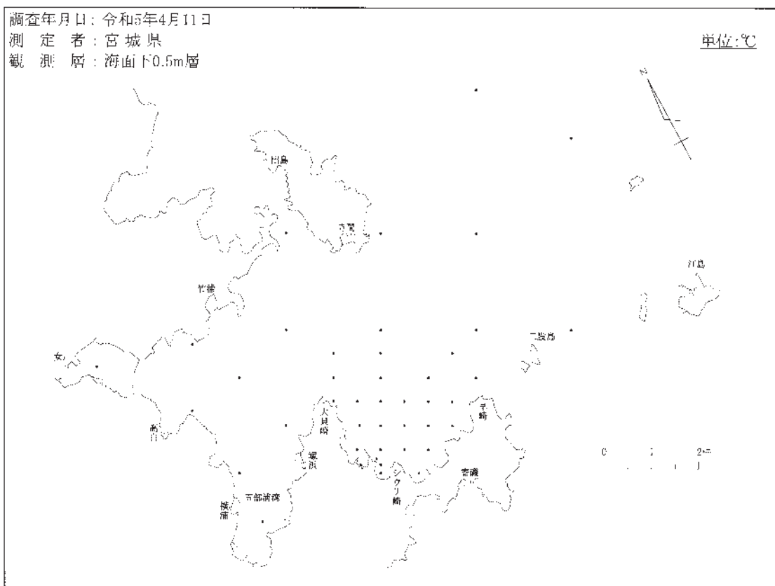
図-2-(2) 等温線
