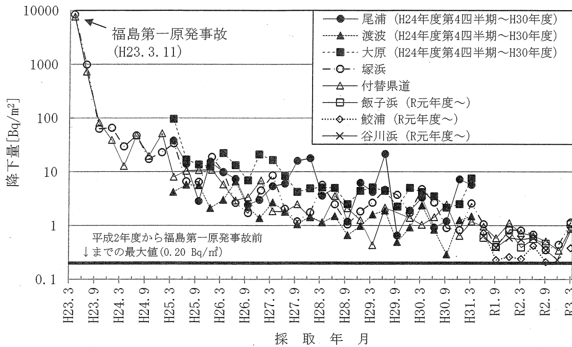
図-5 Cs-137の四半期間降下量の推移
