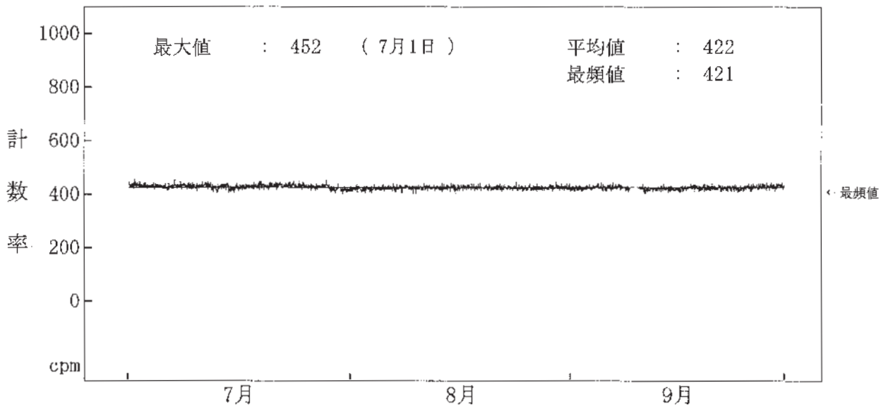
図一 2 - 1 4 海水(放水)中の全ガンマ線計数率監視結果(2号機放水口モニター)
