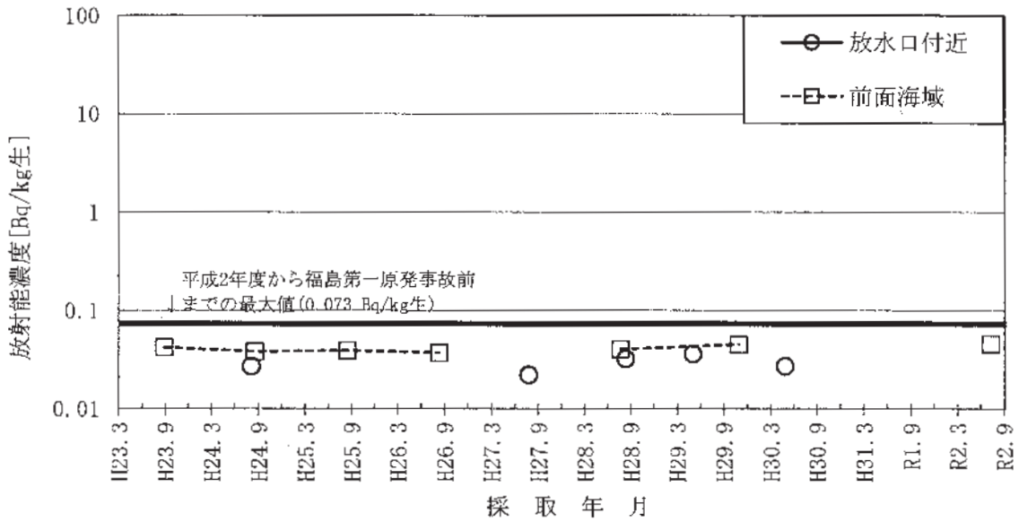
図-2-3 2 アラムのSr-90濃度の推移
