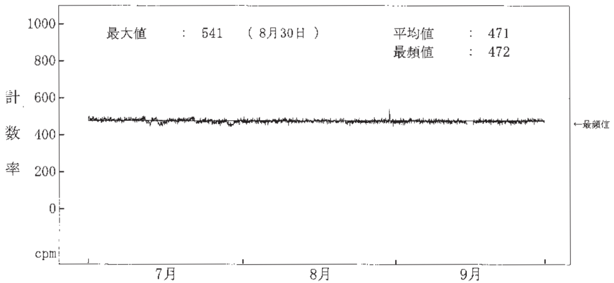
図一 2 - 1 5 海水(放水)中の全ガンマ線計数率監視結果(3号機放水口モニター)
