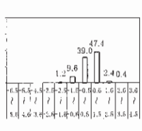
St.9(浮上点付近)とSt.12(2号機取水口)との水温較差
