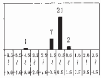
St.9(浮上点付近)とSt.12(2号機取水口)との水温較差
