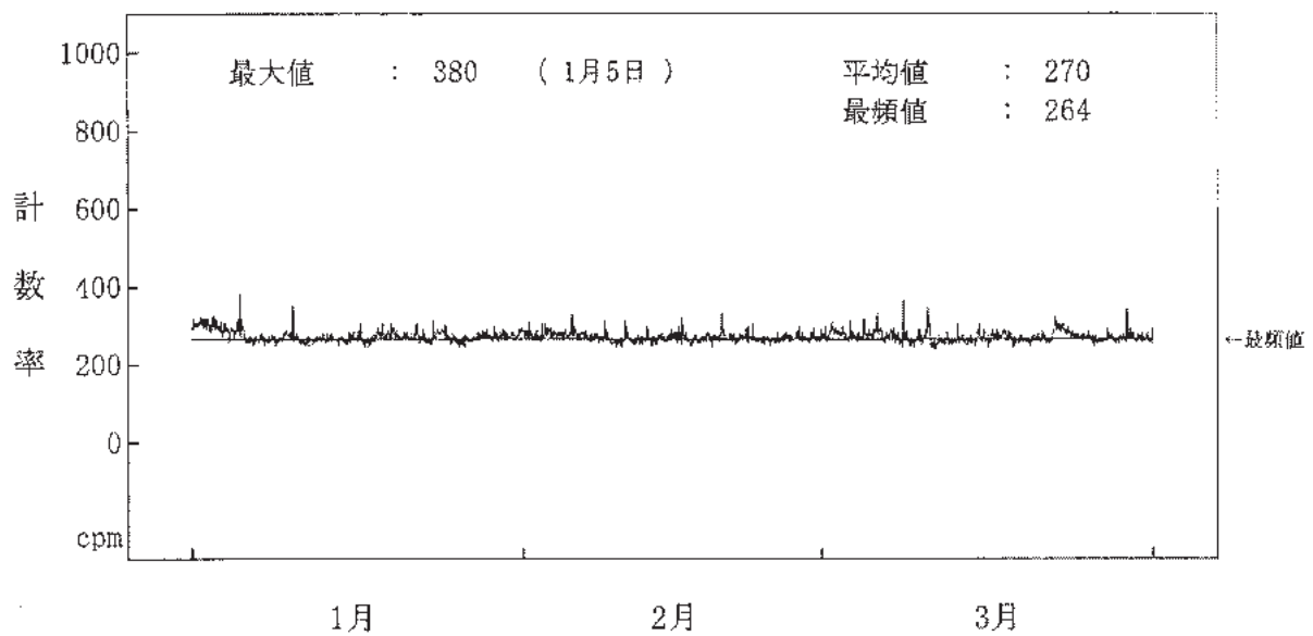
図-2-8 海水(放水)中の全ガンマ線計数率監視結果(1号機放水口モニター(A)) (注) 1月14日の欠測は、構内配電線の停電作業によるものである。
