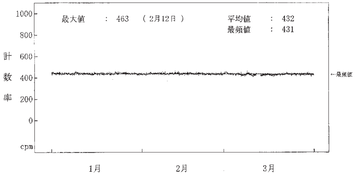
図-2-10 海水(放水)中の全ガンマ線計数率監視結果(2号機放水口モニター) (注) 3月12日～13日の欠測は、定期点検によるものである。
