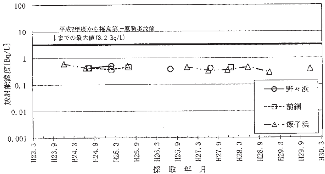
図-2-22 陸水のH-3濃度の推移
