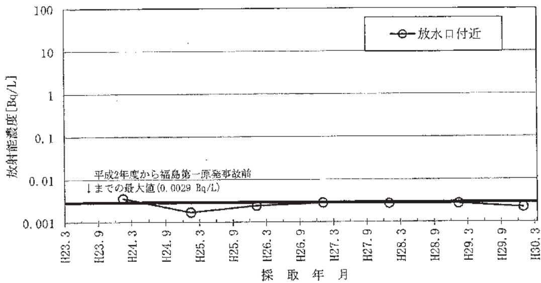
図-2-21 海水のSr-90濃度の推移
