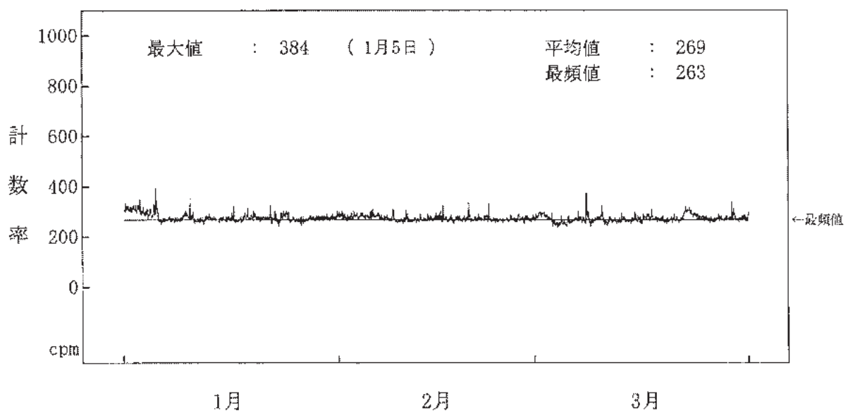
図-2-9 海水(放水)中の全ガンマ線計数率監視結果(1号機放水口モニター(B)) (注) 1月14日の欠測は、構内配電線の停電作業によるものである。
