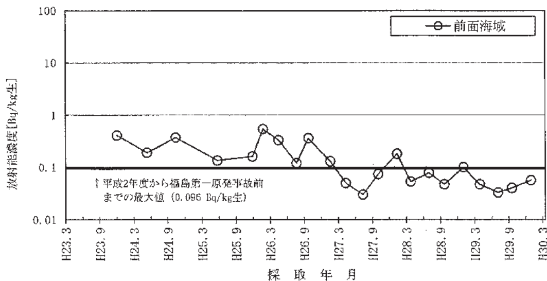
図-2-20 ムラサキガイのCs-137濃度の推移
