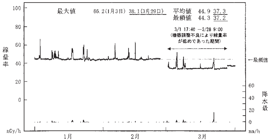
図-2-3 空間ガンマ線線量率監視結果 (青磯局)
