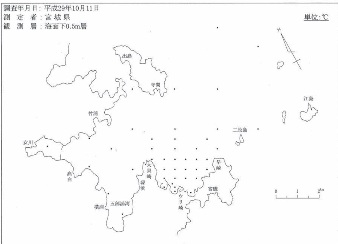
図-2-(2) 等温線
