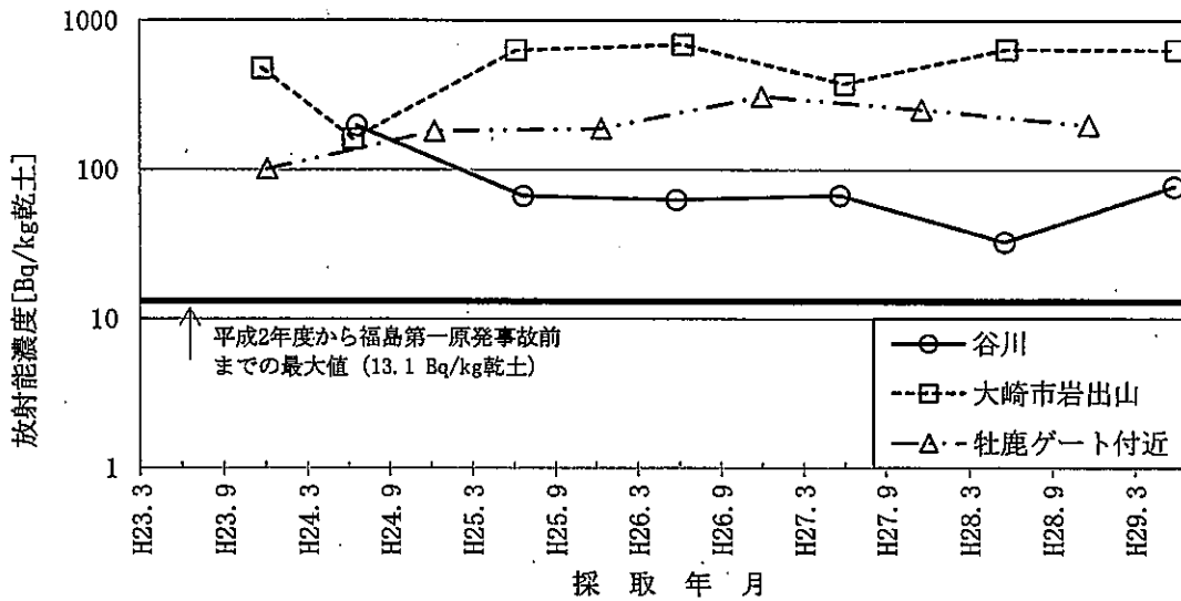
図-2-16 陸士のCs-137濃度の推移
