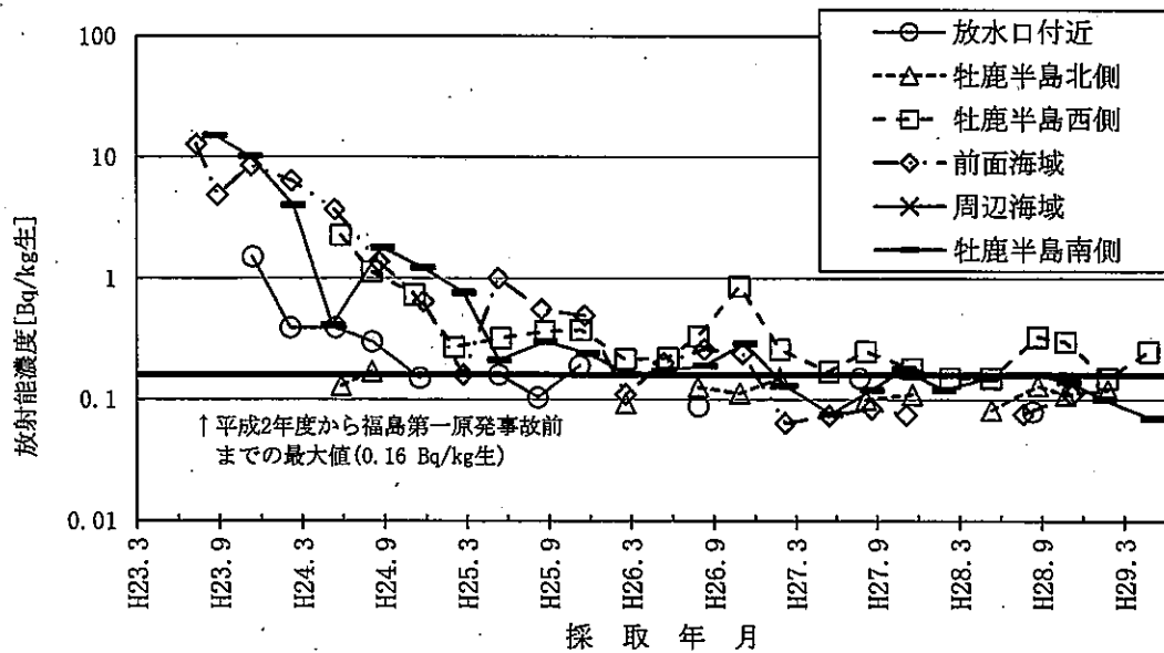
図-2-20 アラメのCs-137濃度の推移
