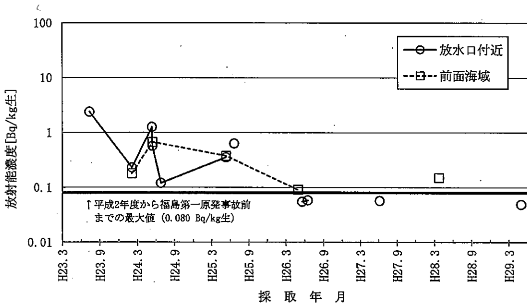
図-2-19 ワカメのCs-137濃度の推移
