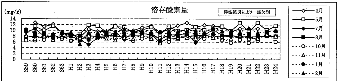
図III-9-(2) 養殖漁場環境点の水質(海面下0.5m層)の月別経年変化 五部浦(St.3)
