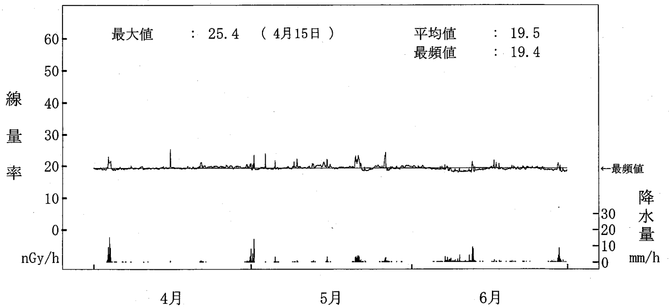
図-2-5 空間ガンマ線線量率監視結果 (寺間局) (注) 下方を鉛で遮へいしたNaI(Tl)検出器により測定した。
