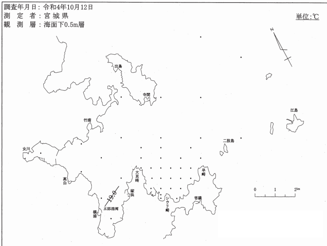
図-2-(2) 等温線
