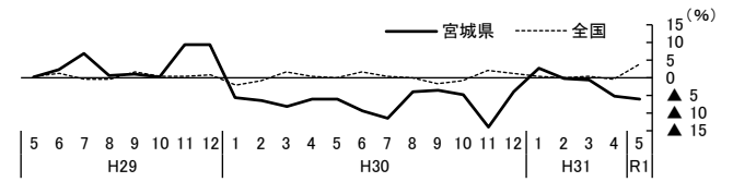
図26：指数
