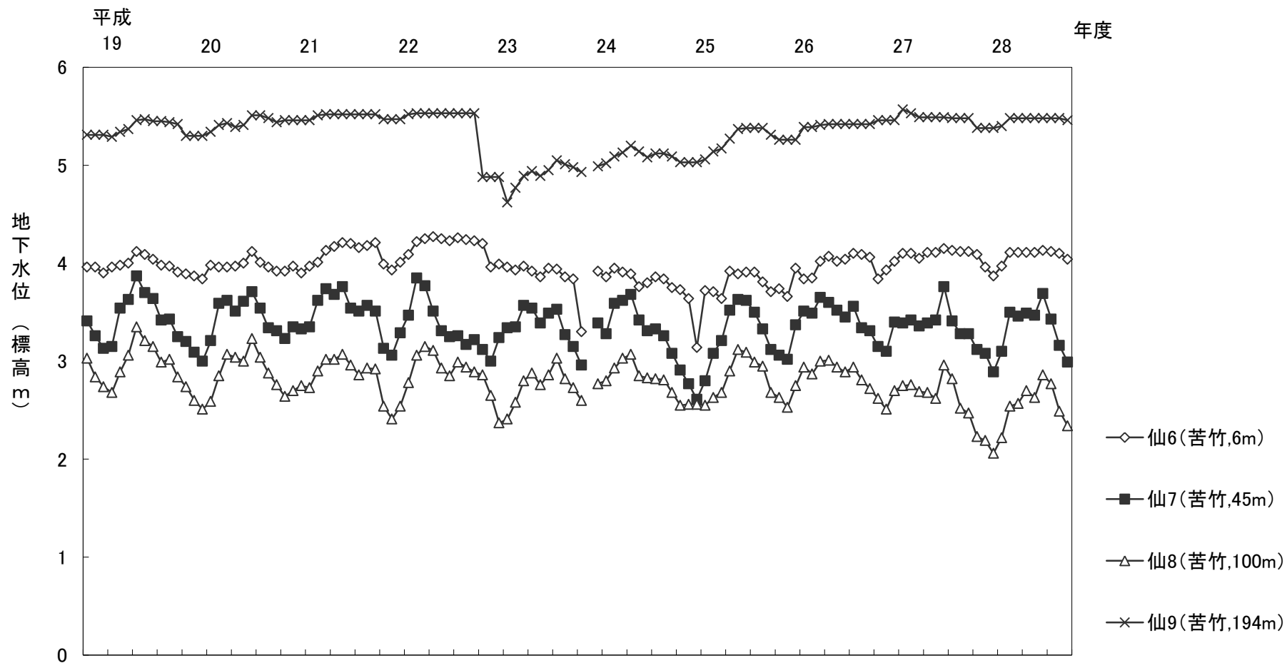
仙台市苦竹地区の地下水位変化図
