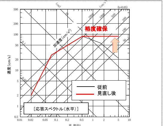
<応答スペクトルの形状見直し>
