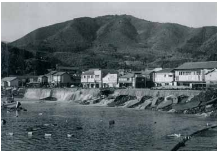
海岸通りの岸壁・被災状況
