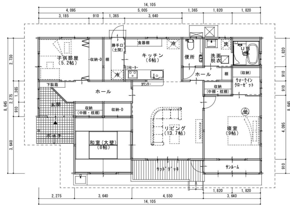
1階平面図
