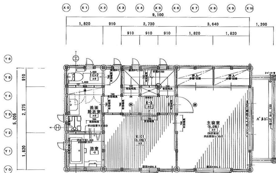
2階平面図
