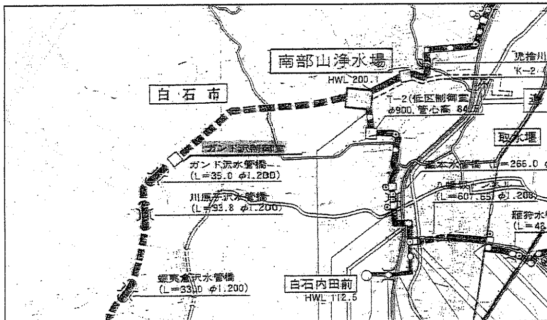
<現場位置図>
