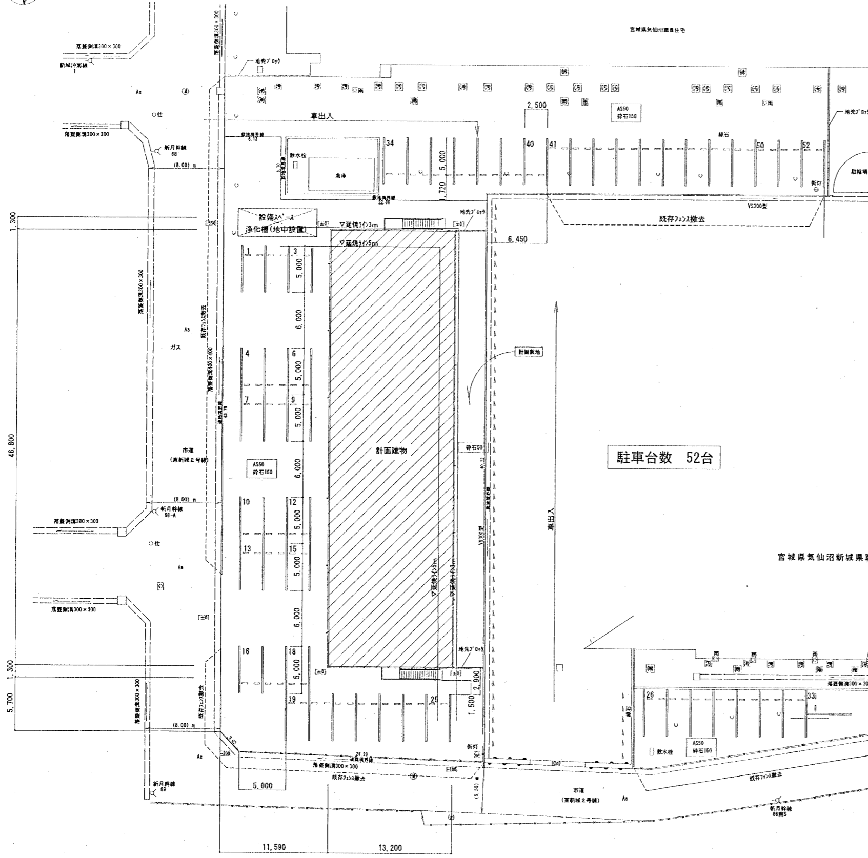
配置図
