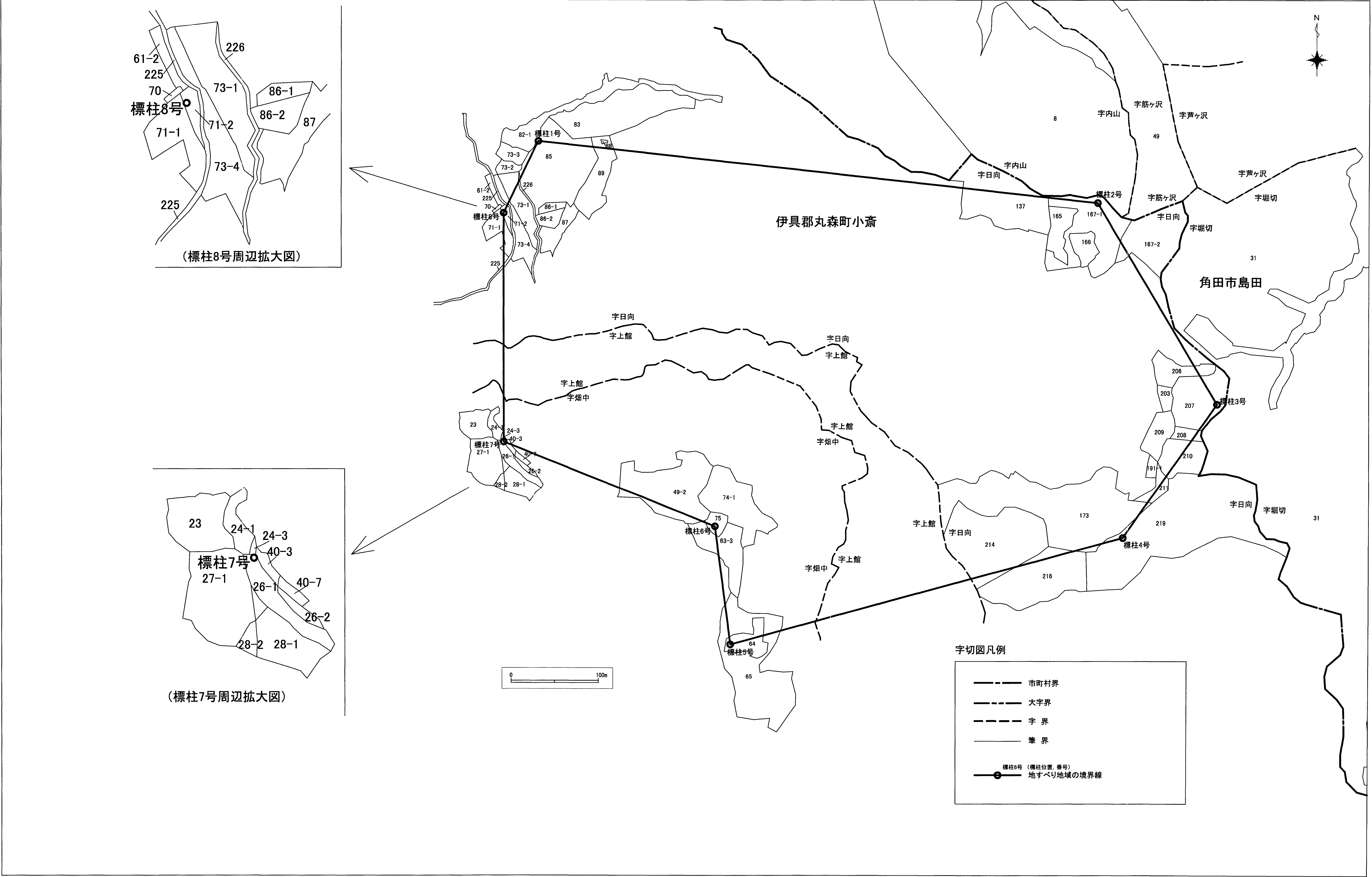
小斎清水 地すべり防止区域 字 切 図 (S=1:2,000)
