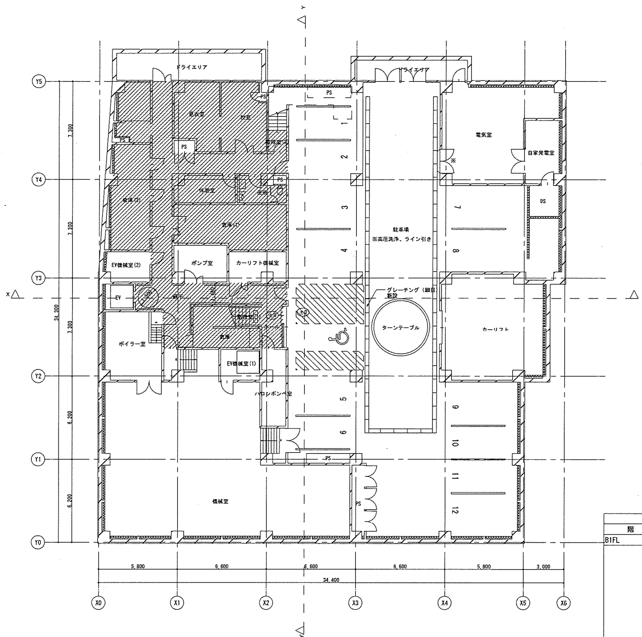
改修 地下1階平面図 1:100
