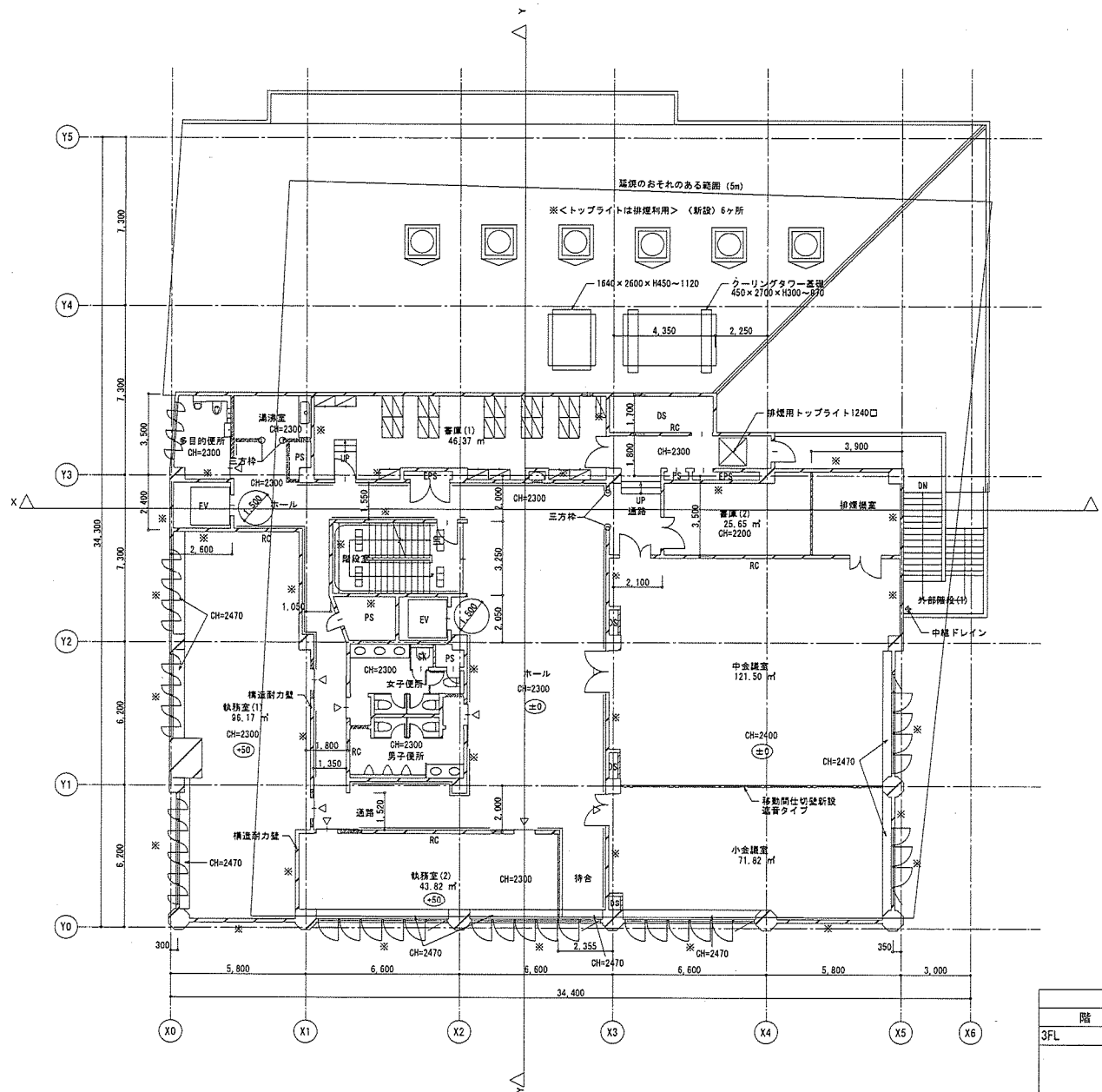
改修 3階平面図 1:100 ※ 真空ガラスに交換
