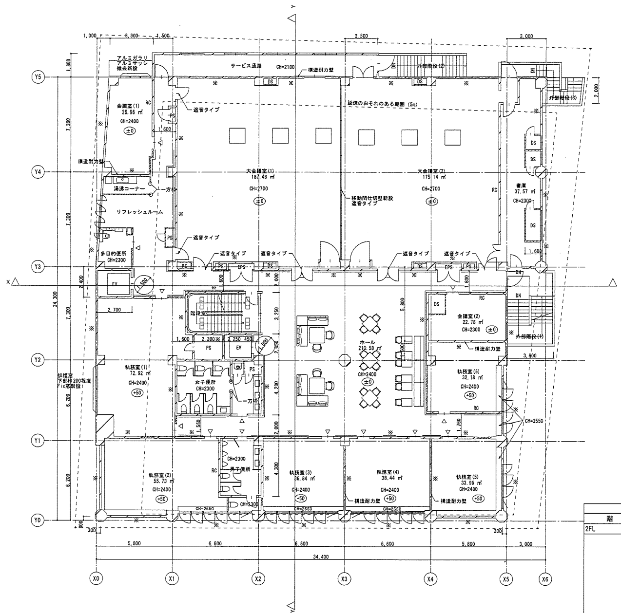
改修 2階平面図 1:100 ※ 真室ガラスに交換
