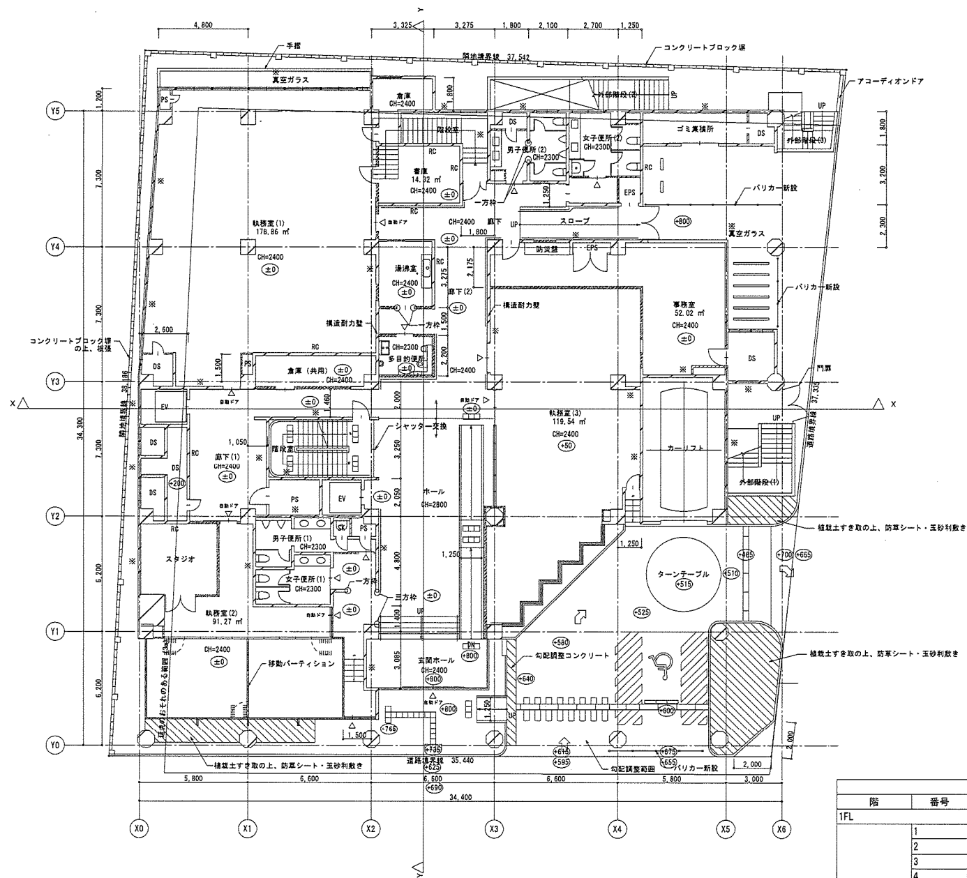
改修 1階平面図 1:100
