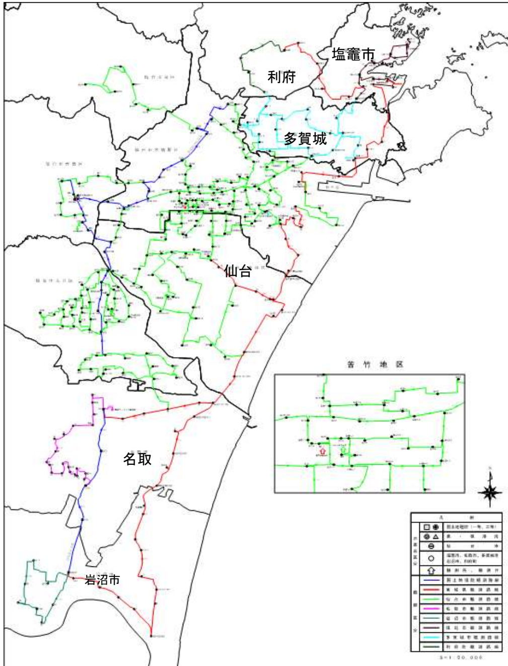
この地図は、国土地理院長の承認を得て、同院発行の5万分の1地形図を複製したもので ▲図2-4-3-1 仙台平野地域水準測量観測路線
