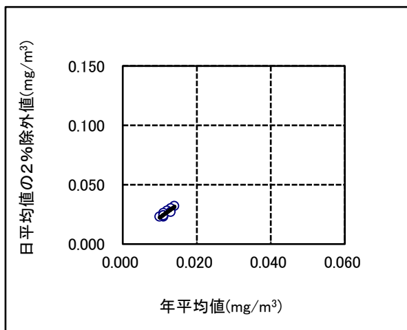
(自排局 SPM)
