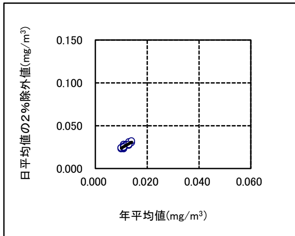
(一般局 SPM)
