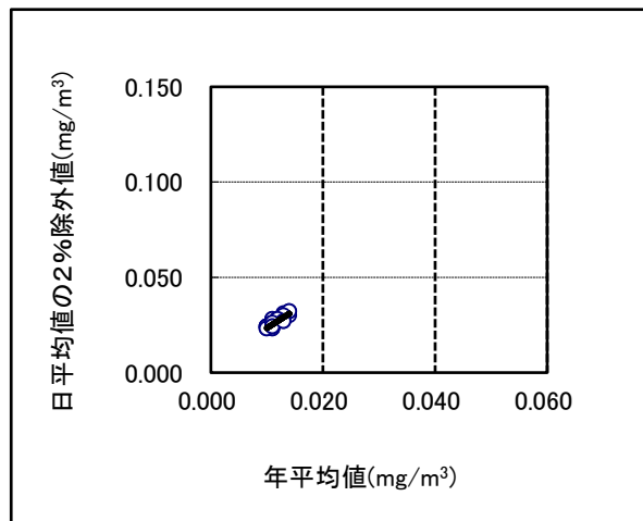
(全局 SPM)
