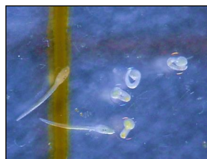
図5 マボヤ幼生
