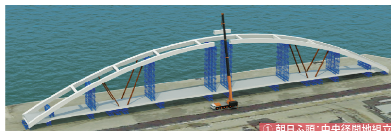
① 朝日ふ頭: 中央径間地組立
