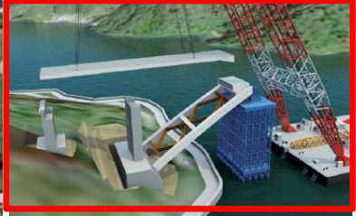
⑤⑨ 補剛桁架設
