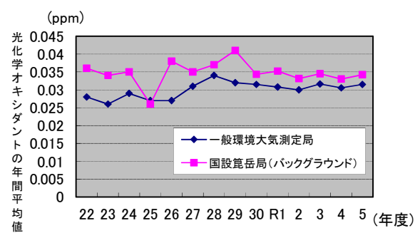
光化学オキシダントの年間値の推移
