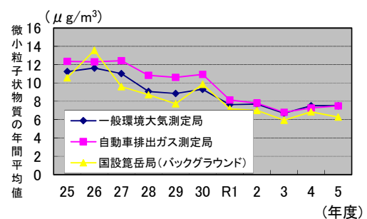
微小粒子状物質の年間平均値の推移
