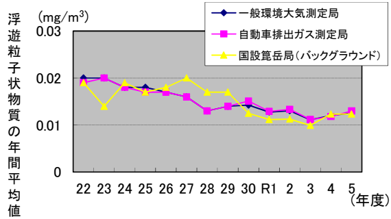
浮遊粒子状物質の年間平均値の推移
