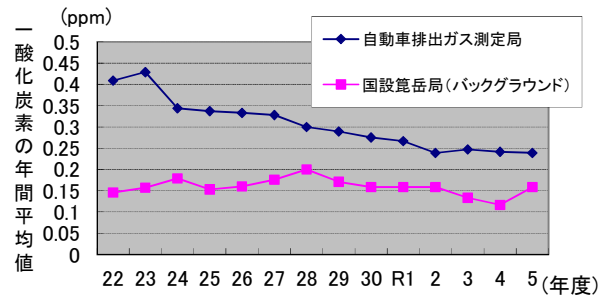
一酸化炭素の年間平均値の推移
