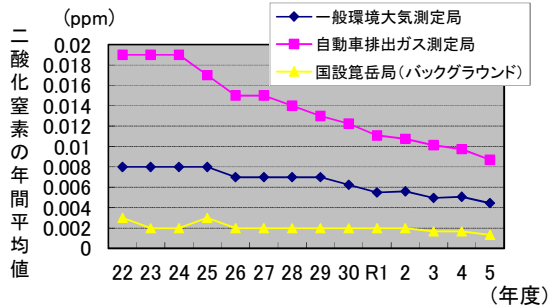
二酸化窒素の年間平均値の推移
