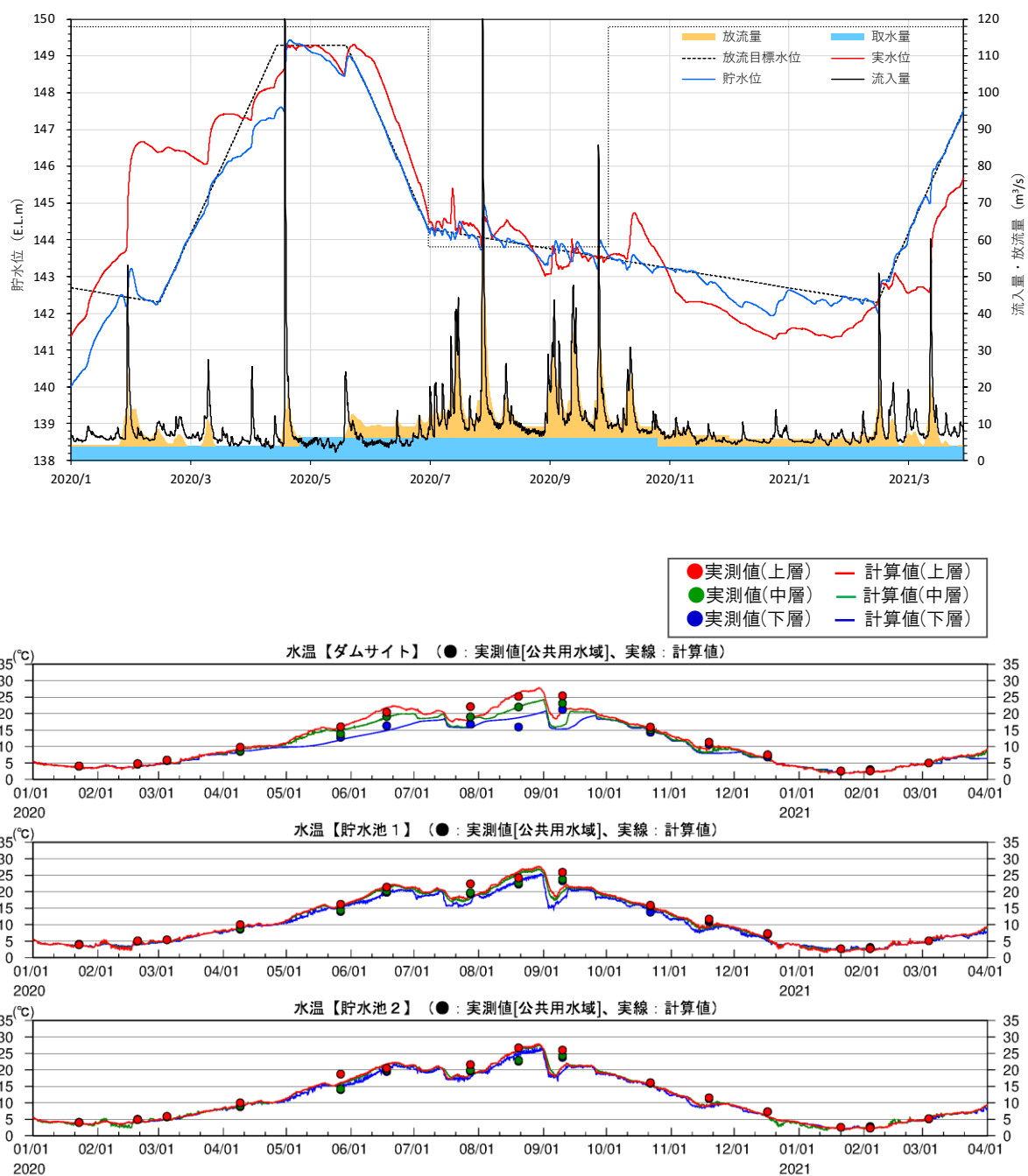
図 2-27(4) 将来シナリオのダム運用ルールに基づく貯水位・放流量・水温試算結果(2020 年)
