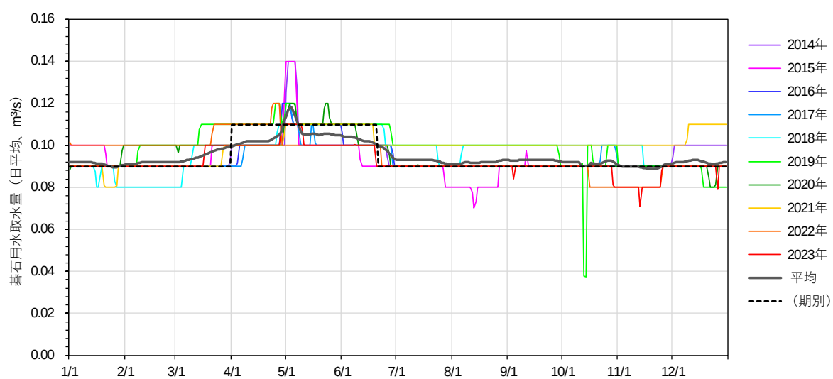
図 2-22 基石用水取水量
