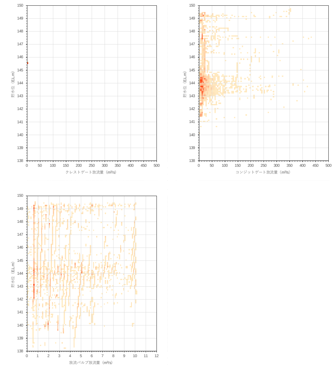
図 2-18 各ゲート・バルブからの放流量と貯水位の関係
