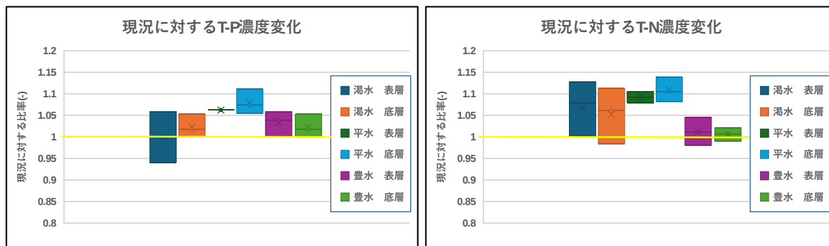
図 2-32(2) 現況に対する予測結果の濃度変化 (T-P, T-N)
