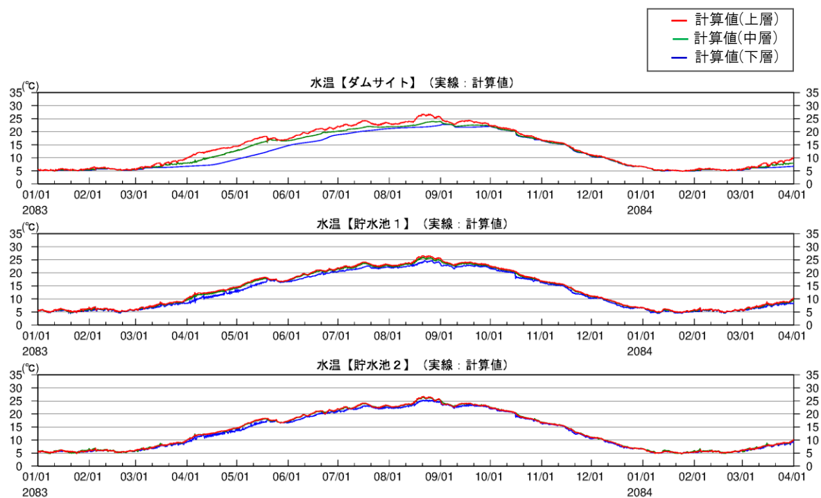
図 2-30(5) 将来シナリオにおける釜房ダム水質予測結果(平水年②:2083_GF_m105)
