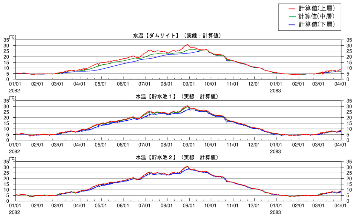
図 2-30(6) 将来シナリオにおける釜房ダム水質予測結果(平水年③:2082_MI_m105)
