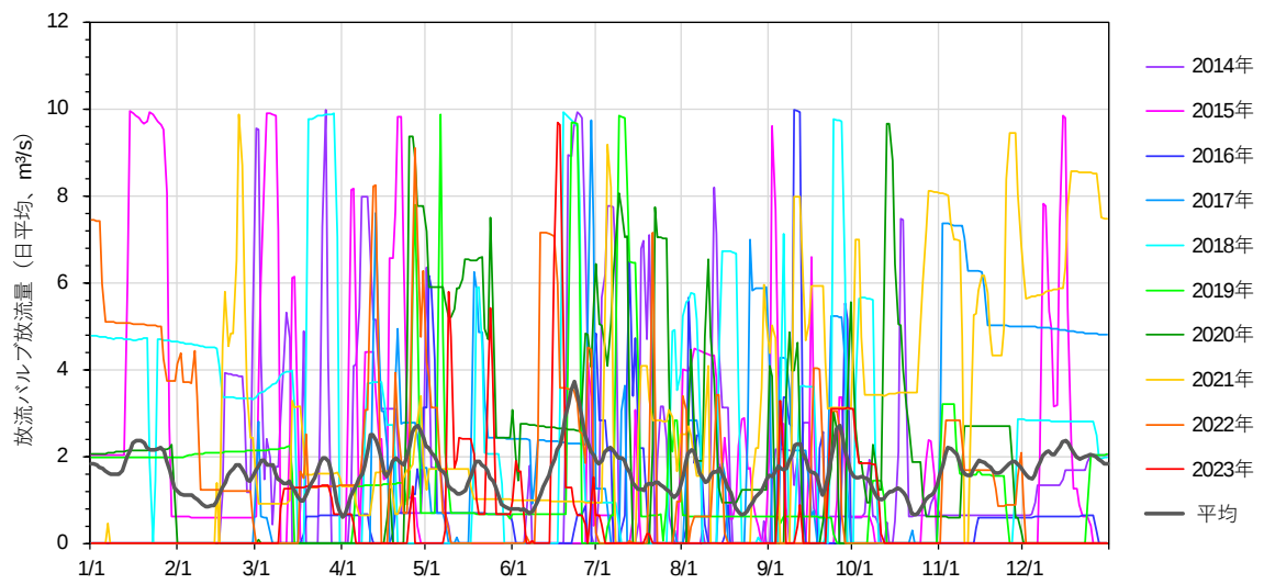
図 2-16 放流バルブ放流量
