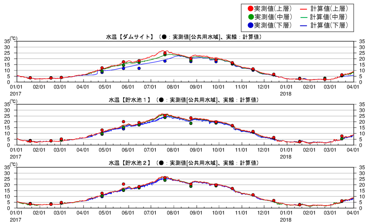
図 2-27(1) 将来シナリオのダム運用ルールに基づく貯水位・放流量・水温試算結果(2017 年)
