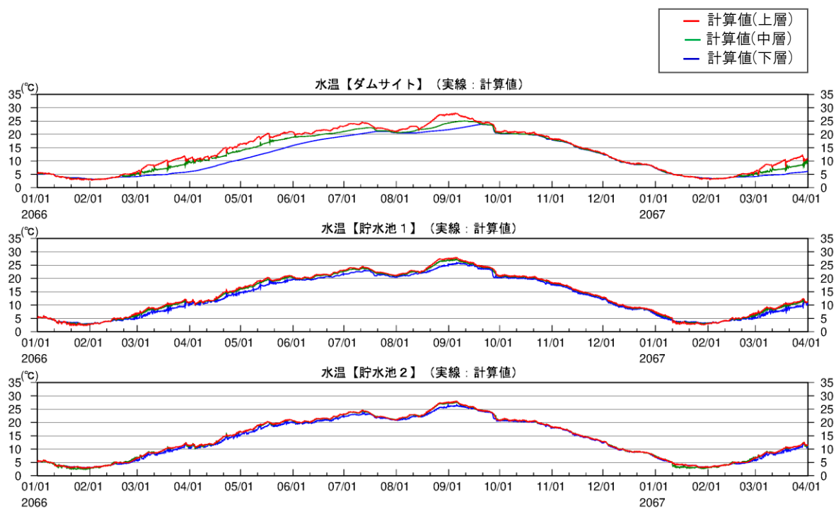
図 2-30(2) 将来シナリオにおける釜房ダム水質予測結果(渇水年②: 2066_CC_m105)
