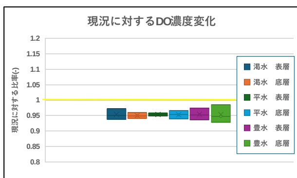
図 2-32(3) 現況に対する予測結果の濃度変化 (DO)
