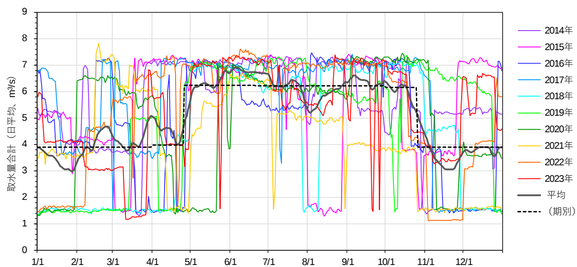
図 2-23 合計取水量
