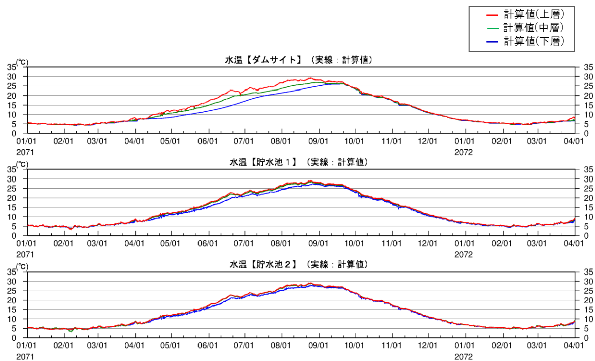
図 2-30(3) 将来シナリオにおける釜房ダム水質予測結果(渇水年③: 2071_CC_m105)
