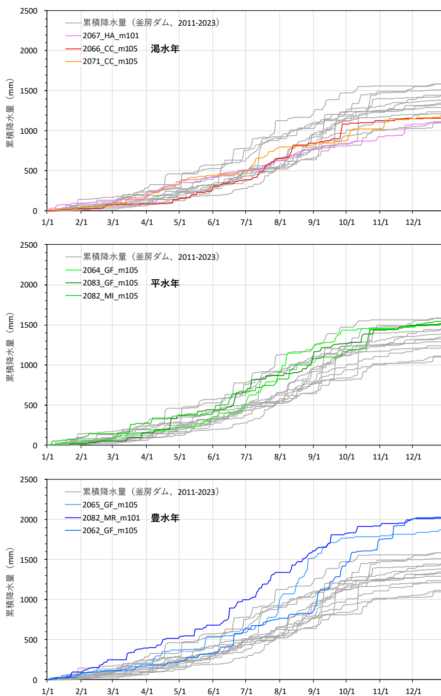
図 2-5 将来シナリオにおける累積降水量
