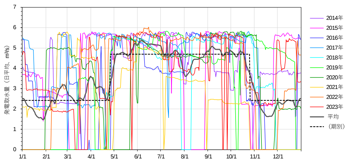
図 2-20 発電取水量
