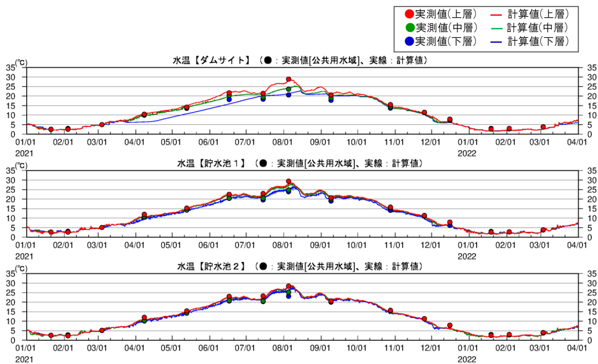
図 2-27(5) 将来シナリオのダム運用ルールに基づく貯水位・放流量・水温試算結果(2021 年)
