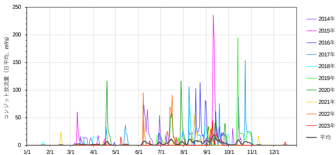
図 2-15 コンジットゲート放流量
