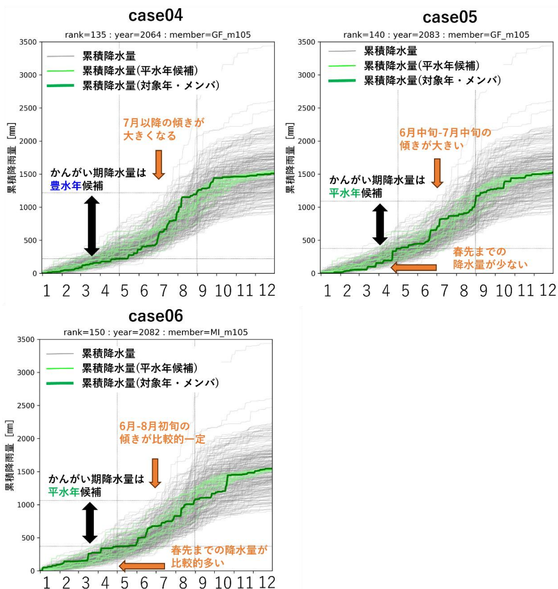
図 2-3 選択した平水年シナリオの累積降水量
