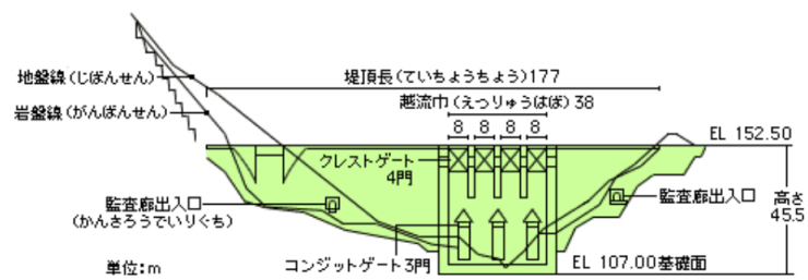
図 2-19 （参考）釜房ダムの堤体断面図・堤体下流面図
