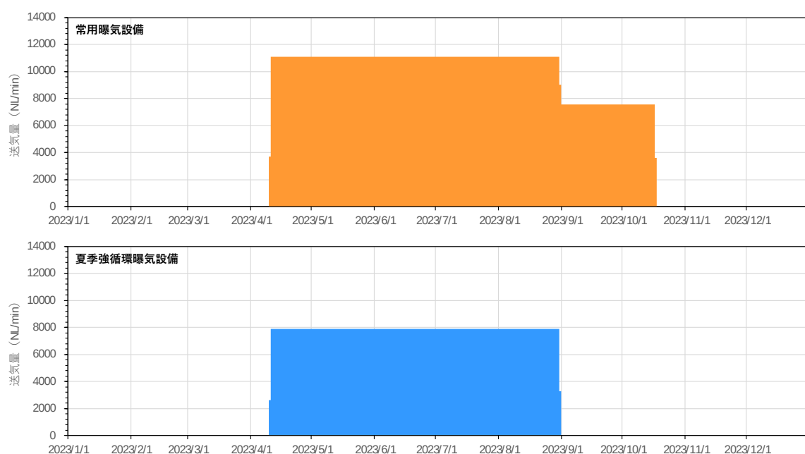
図 2-25(7) 曝気装置運用状況(2023 年)
