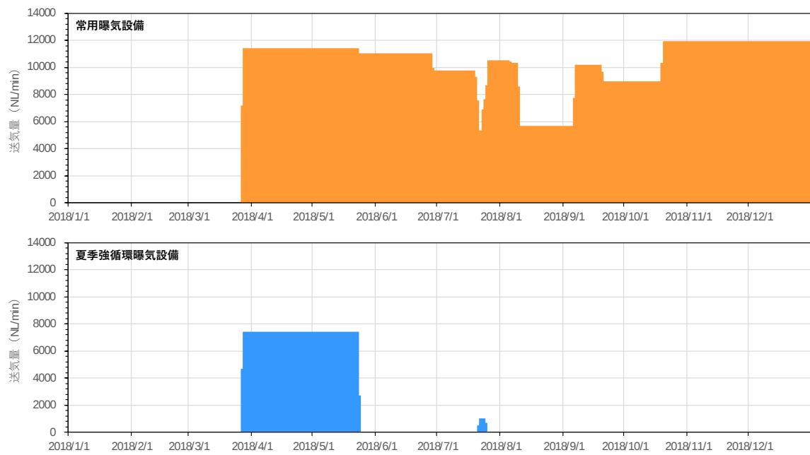
圖 2-25(2) 曝氣裝置運用狀況(2018 年)
