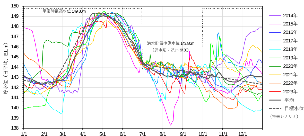
図 2-13 釜房ダムの貯水位
