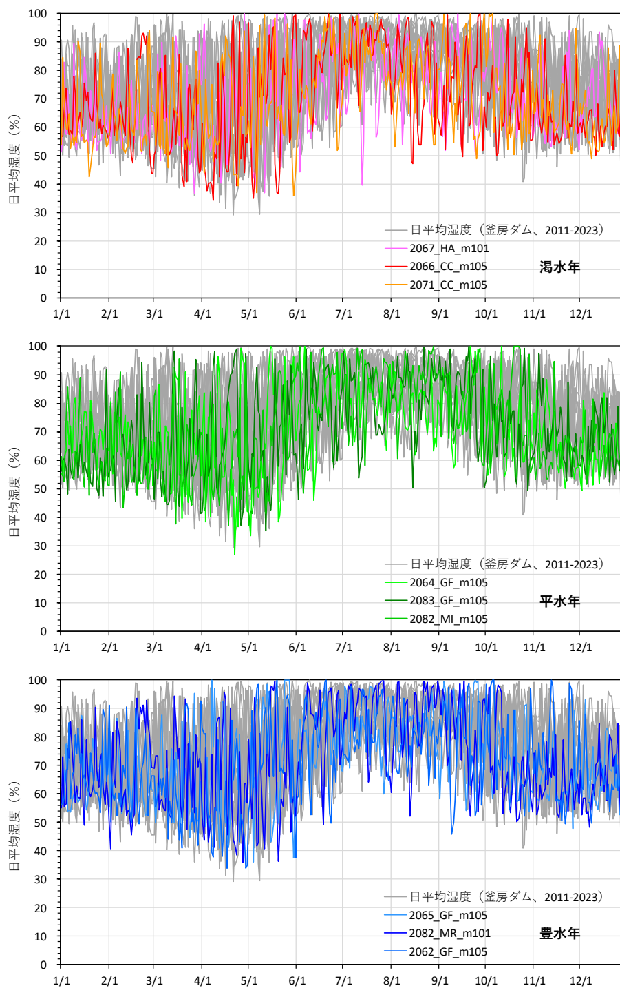
図 2-7 将来シナリオにおける日平均湿度
