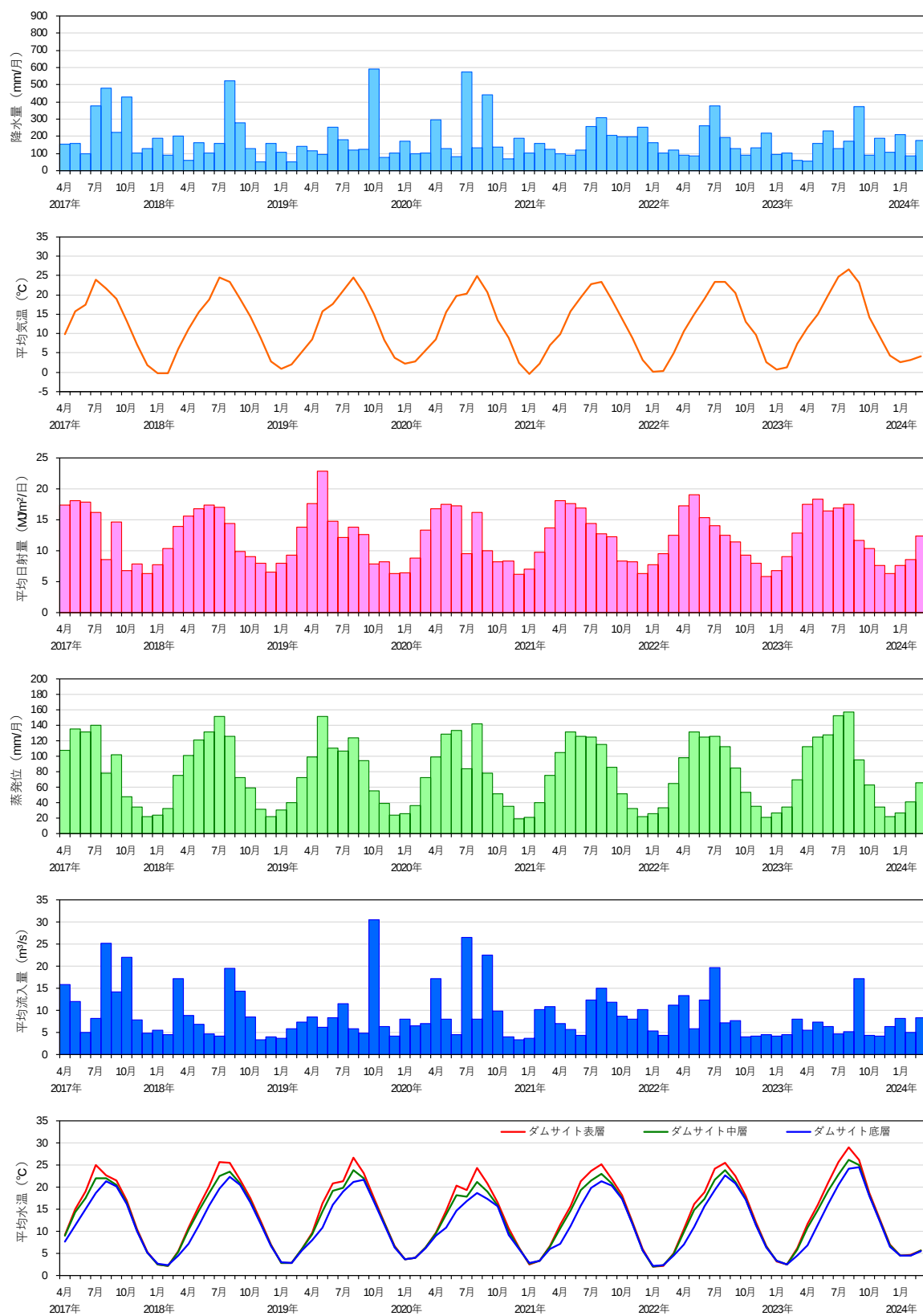
図 2-29(1) 気象・流入条件及び水温計算結果の概要(現況)
