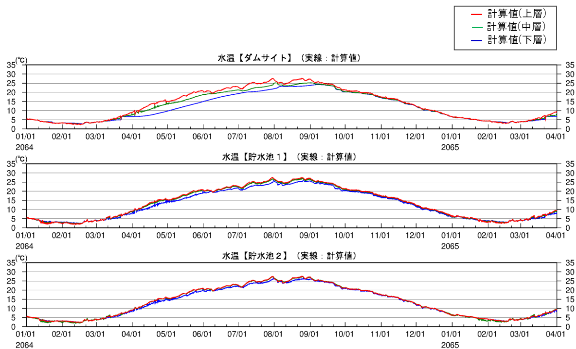
図 2-30(4) 将来シナリオにおける釜房ダム水質予測結果(平水年①:2064_GF_m105)
