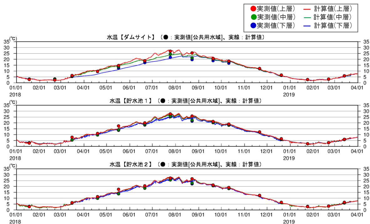
図 2-27(2) 将来シナリオのダム運用ルールに基づく貯水位・放流量・水温試算結果(2018 年)
