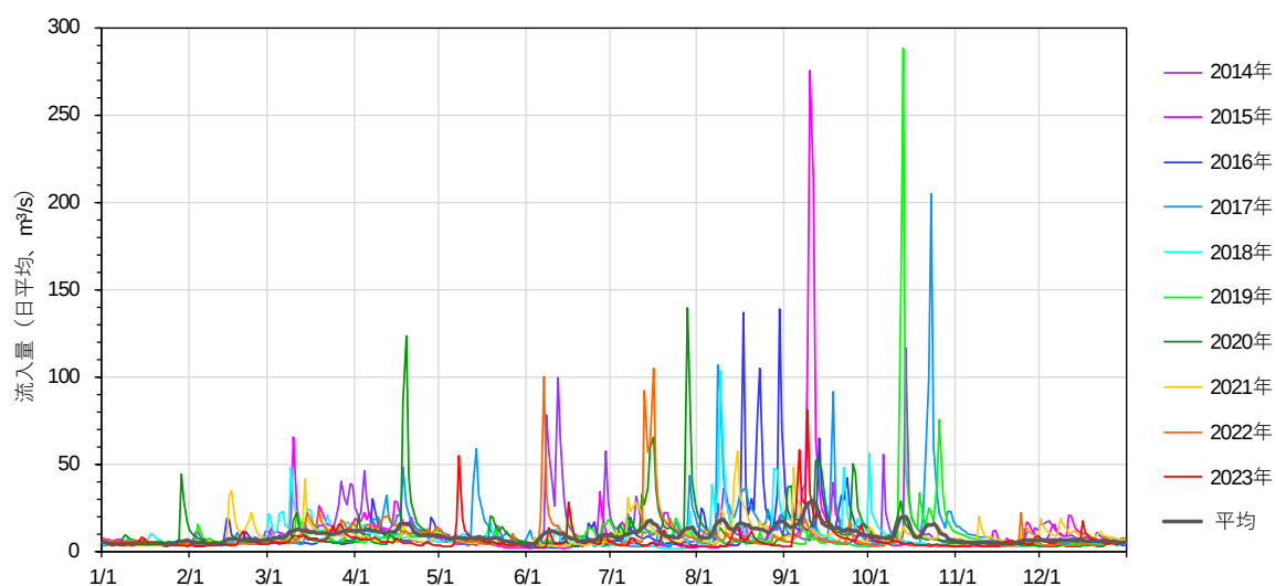
図 2-12 釜房ダムの流入量
