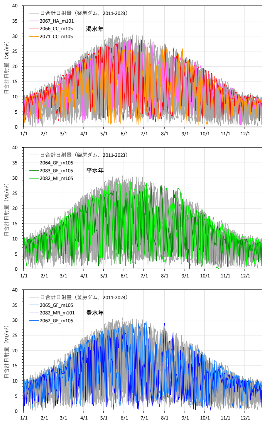
図 2-9 将来シナリオにおける日合計日射量
