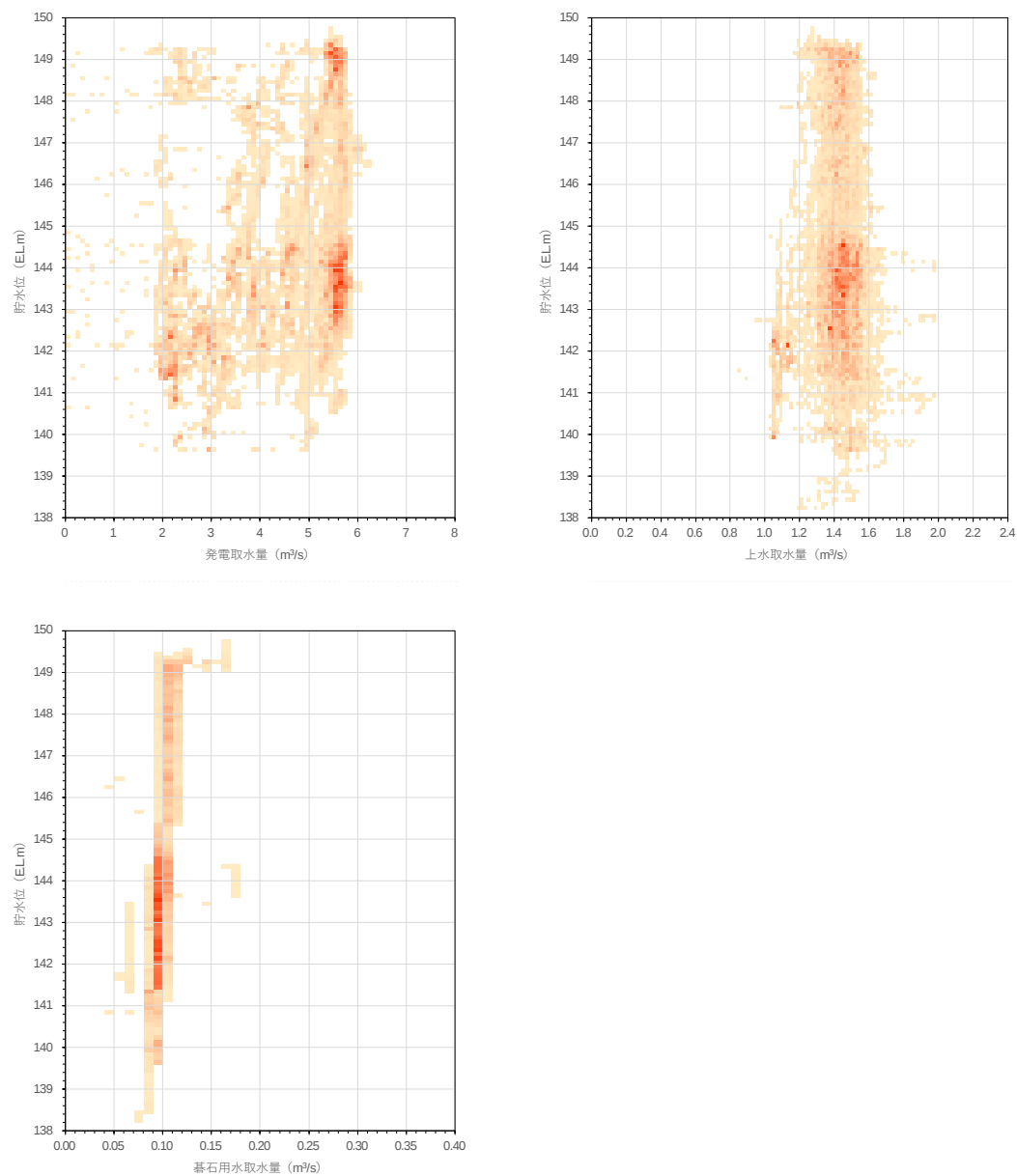
図 2-24 各取水量と貯水位の関係
