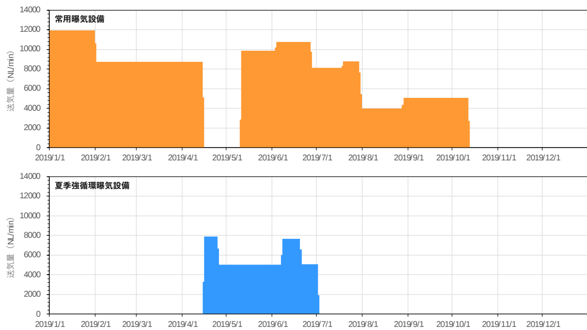
図 2-25(3) 曝氣装置運用状況(2019 年)
