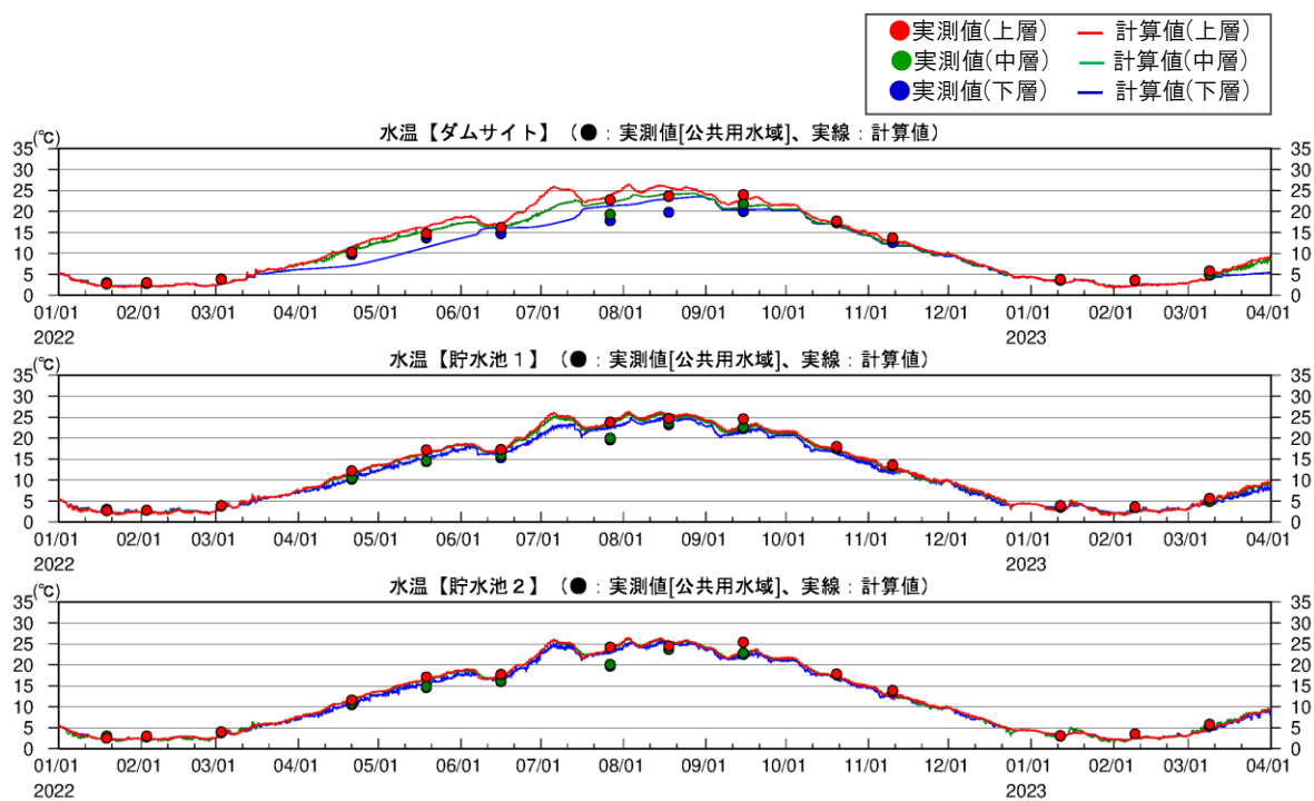
図 2-27(6) 将来シナリオのダム運用ルールに基づく貯水位・放流量・水温試算結果(2022 年)
