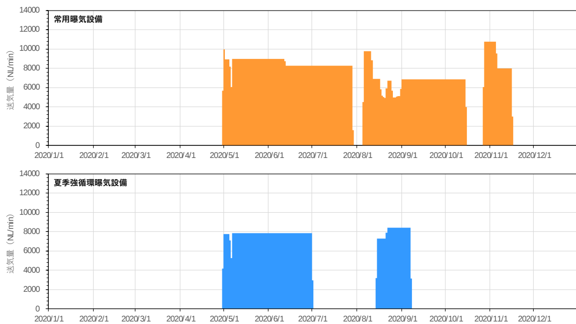
図 2-25(4) 曝氣装置運用状況(2020 年)
