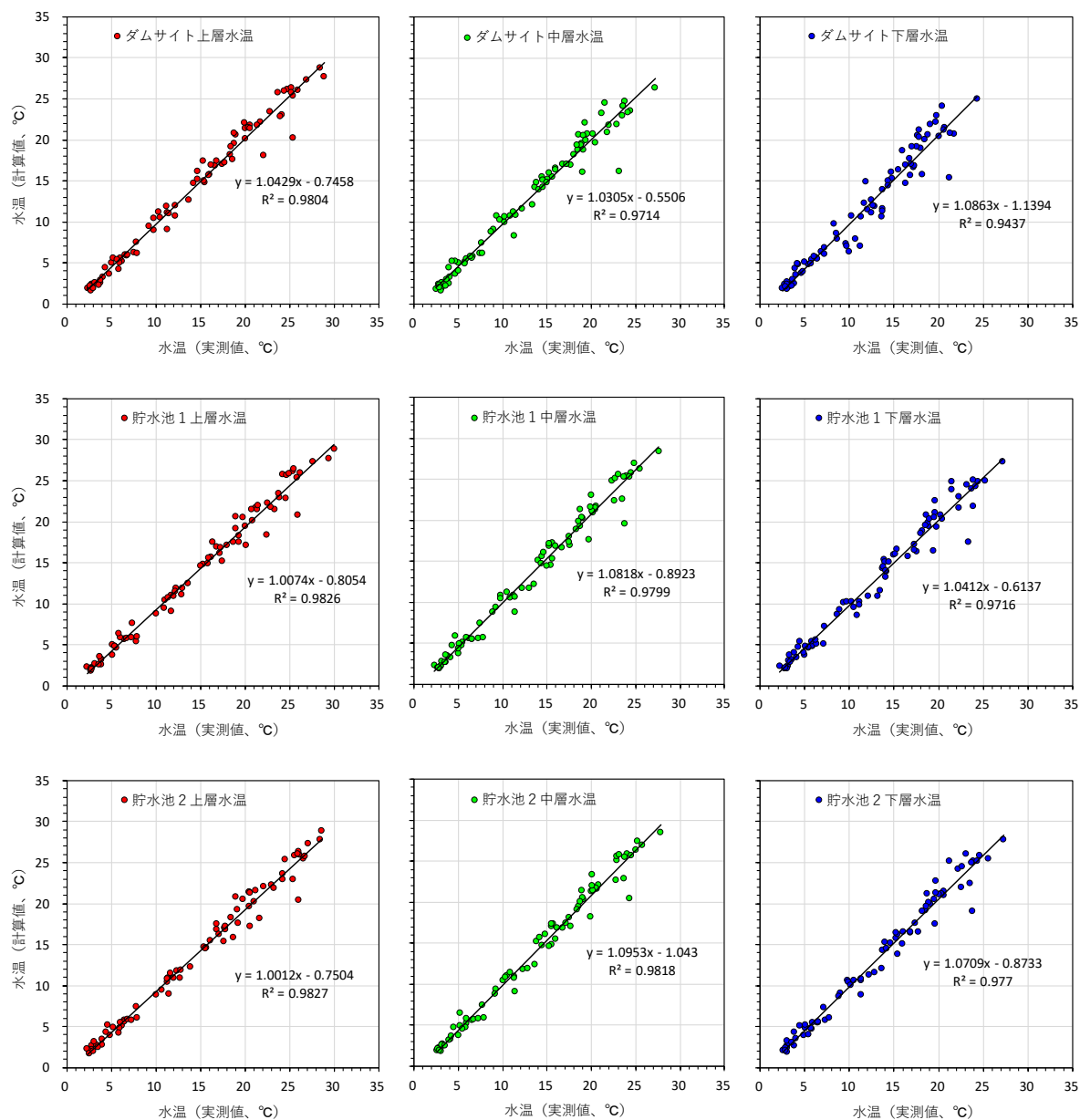
図 2-28 水温の実測値と計算値の比較 平成 29(2017)年度～令和 5 年度 (将来シナリオのダム運用ルールに基づく試算結果)
