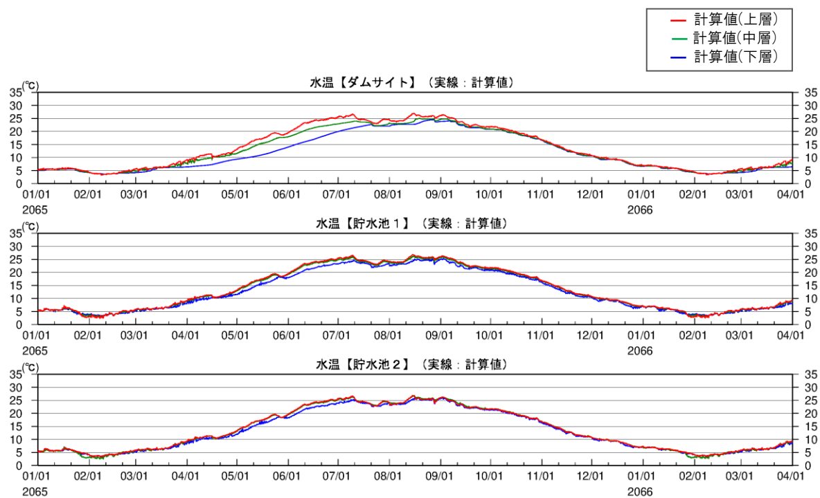
図 2-30(7) 将来シナリオにおける釜房ダム水質予測結果(豊水年①:2065_GF_m105)
