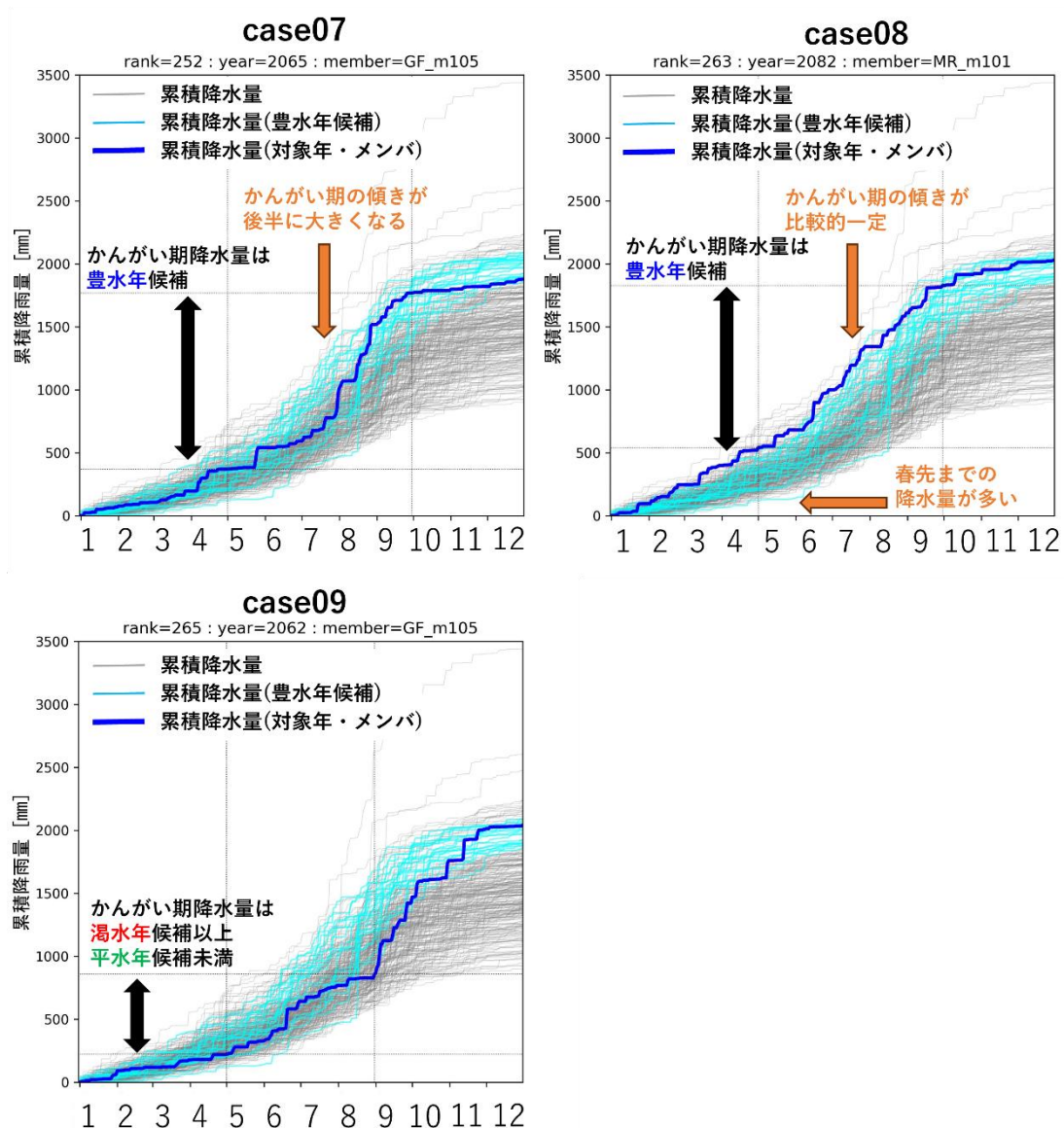
図 2-4 選択した豊水年シナリオの累積降水量
