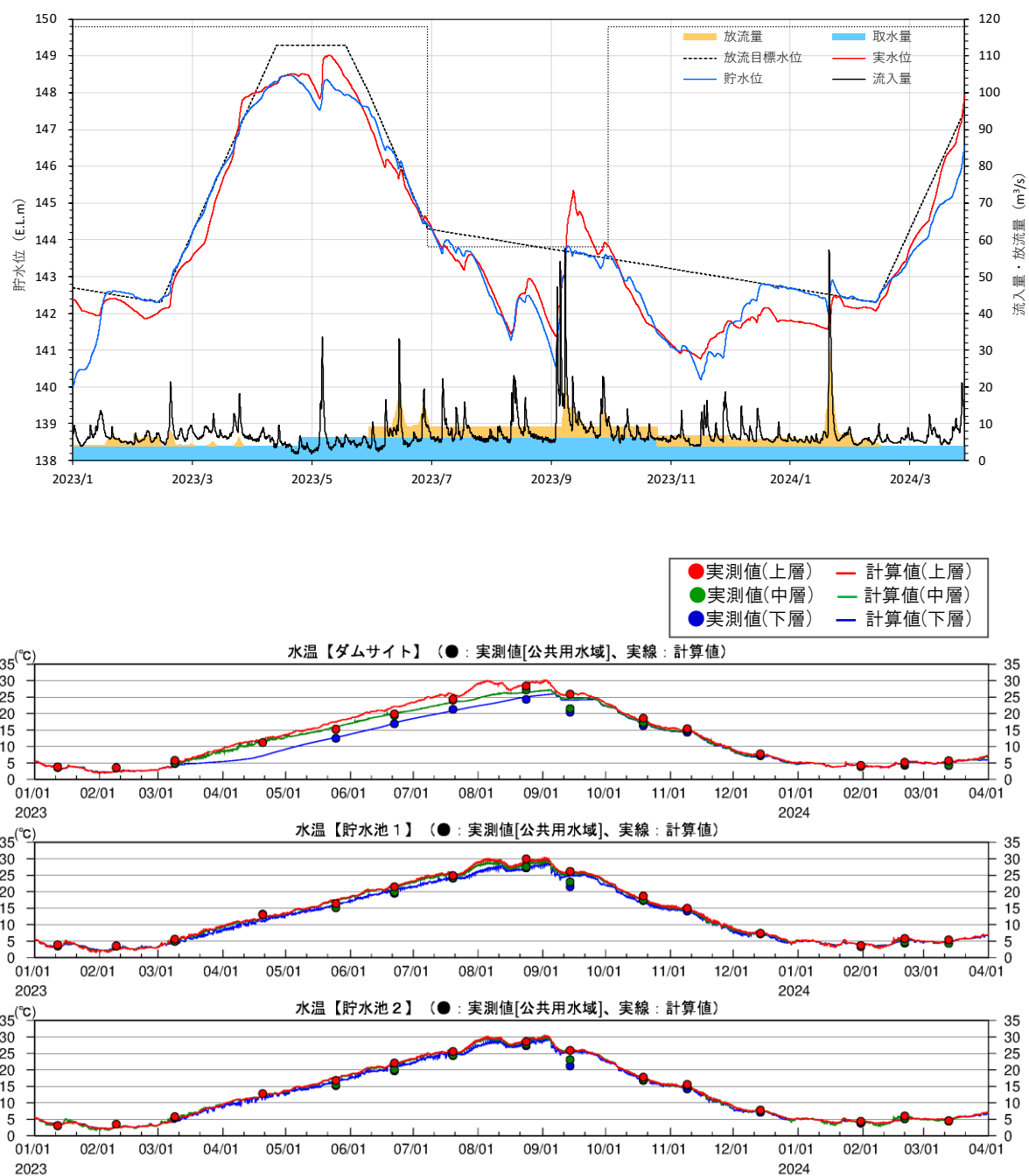
図 2-27(7) 将来シナリオのダム運用ルールに基づく貯水位・放流量・水温試算結果(2023 年)
