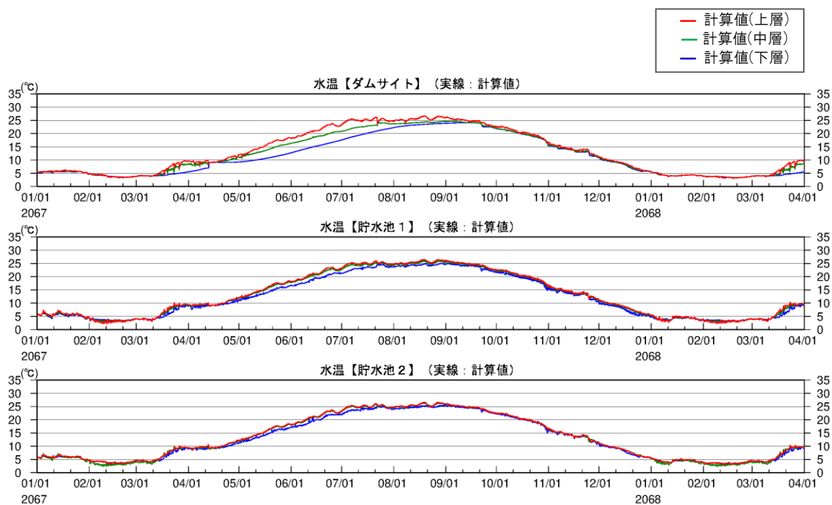
図 2-30(1) 将来シナリオにおける釜房ダム水質予測結果(渇水年①:2067_HA_m101)
