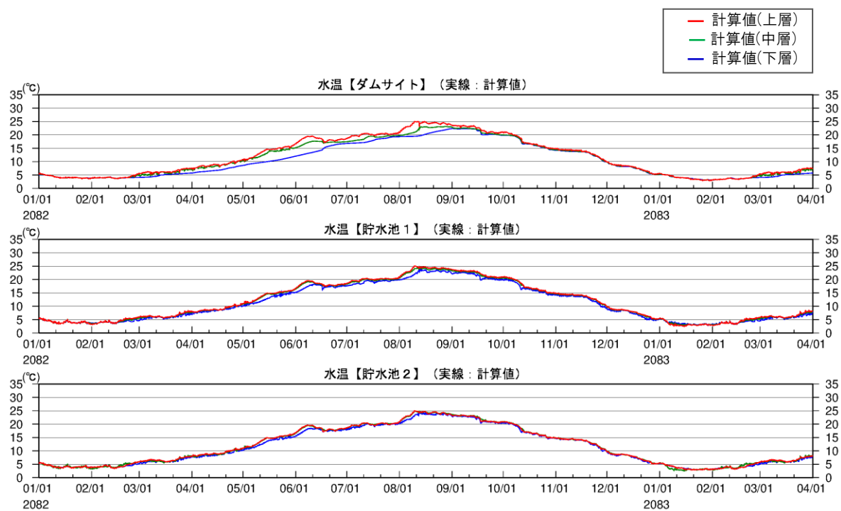
図 2-30(8) 将来シナリオにおける釜房ダム水質予測結果(豊水年②:2082_MR_m101)
