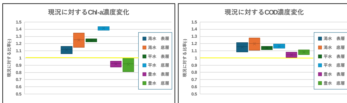
図 2-32(1) 現況に対する予測結果の濃度変化(Chl-a, COD)
