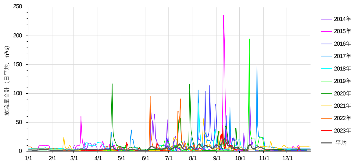
図 2-17 合計放流量
