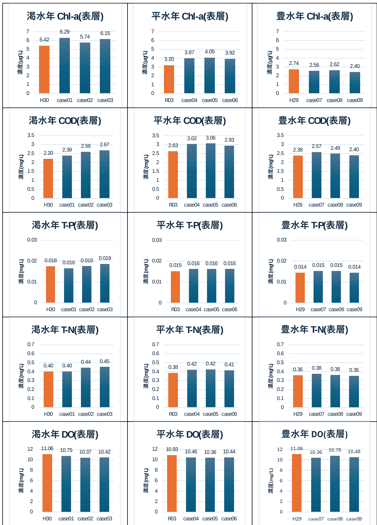
図 2-33(1) 渇水年・平水年・豊水年の現況基準年度と予測結果の濃度(表層)
