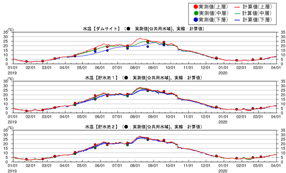
図 2-27(3) 将来シナリオのダム運用ルールに基づく貯水位・放流量・水温試算結果(2019 年)
