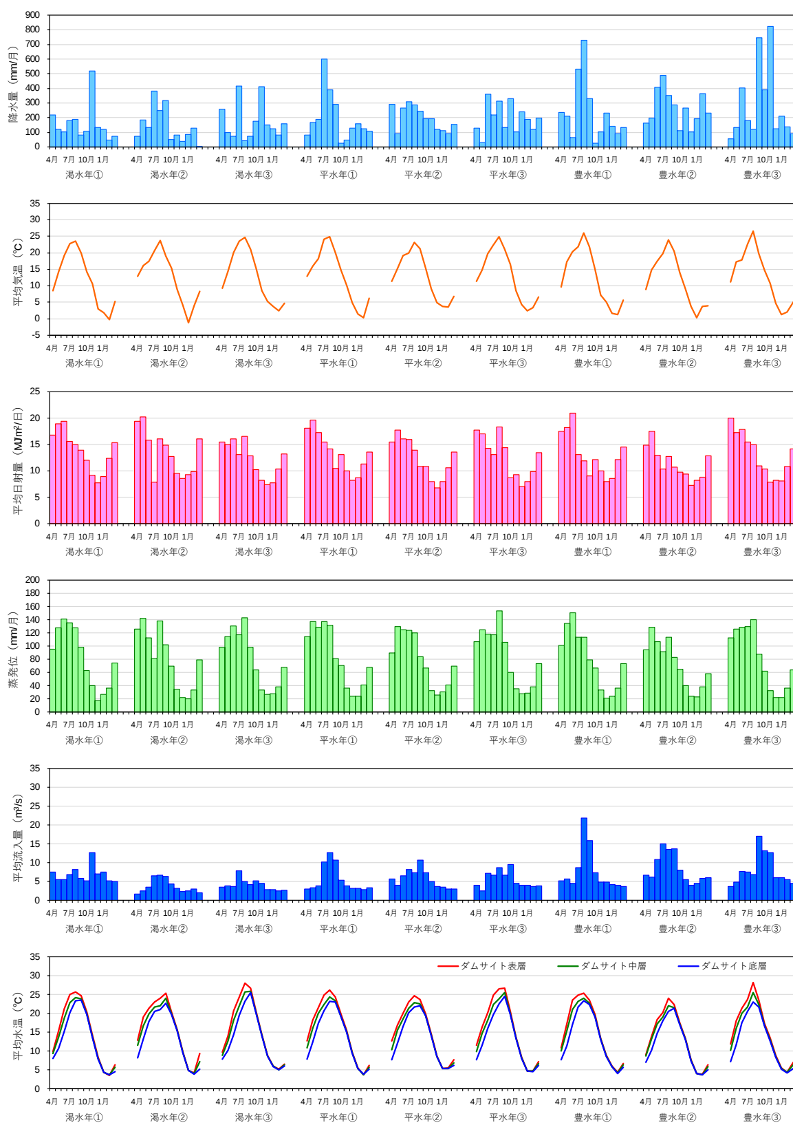
図 2-29(2) 気象・流入条件及び水温計算結果の概要(将来シナリオ)
