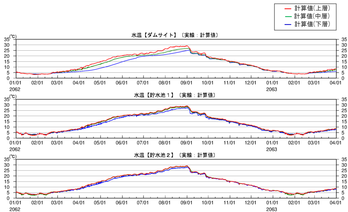
図 2-30(9) 将来シナリオにおける釜房ダム水質予測結果(豊水年③:2062_GF_m105)
