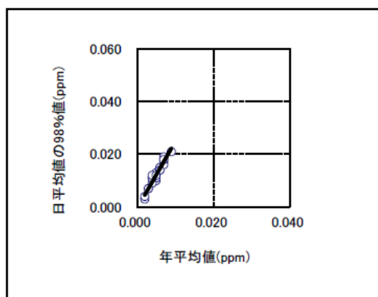
図 6.1.2-7 二酸化窒素の年平均値と日平均値の98%値の相関図
