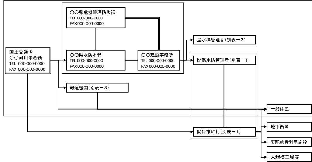
資料 4－5 水防法に基づく水位到達情報（国土交通省発表）の伝達経路等（例） 水防法に定められた水位到達情報の通知・周知は必須であるが、地域防災計画等に基づく手続き等にも留意して伝達経路等を定める。
