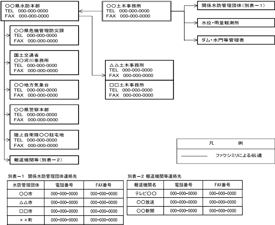
資料 4－14 水防警報（都道府県発表）の伝達経路等（例. 河川）
