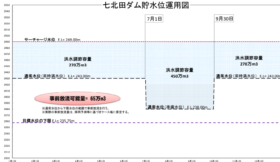
七北田ダム貯水位運用図
