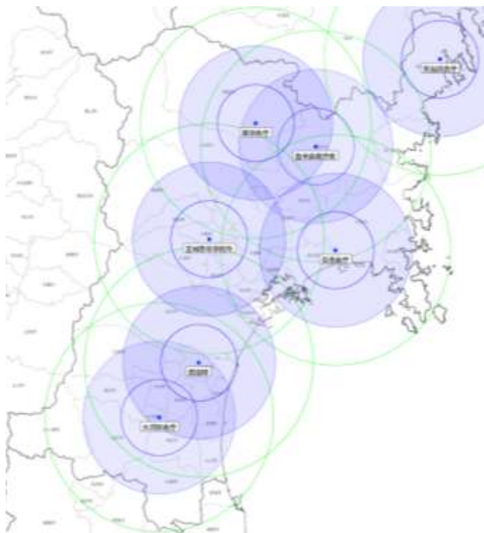
図 8 RTK 基地局の設置場所
