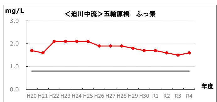
016-53 五輪原橋
