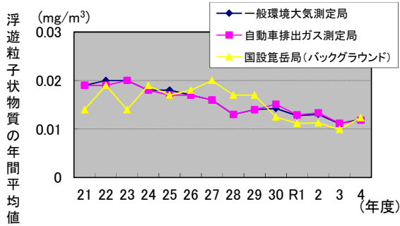
浮遊粒子状物質の年間平均値の推移
