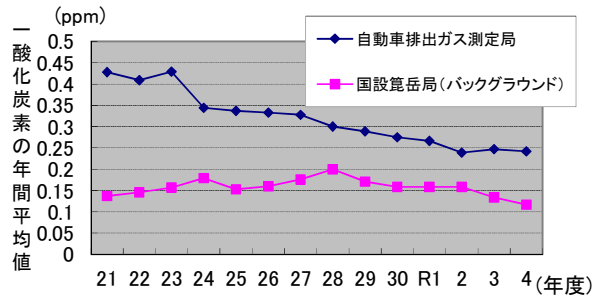
一酸化炭素の年間平均値の推移
