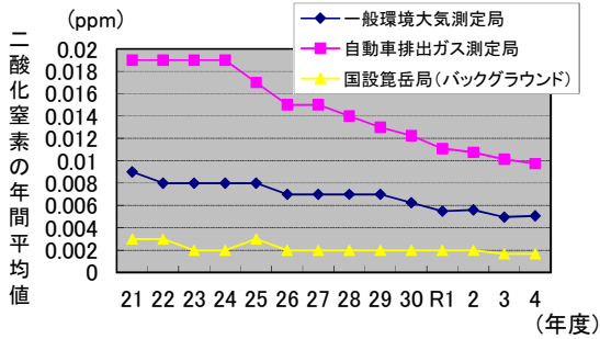
二酸化窒素の年間平均値の推移
