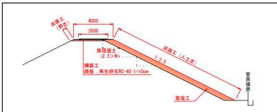
断面図のイメージ (鶴田川)
