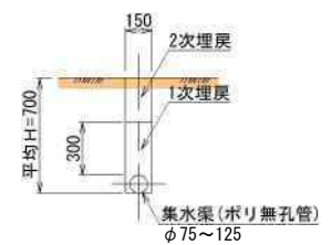
集水渠断面
