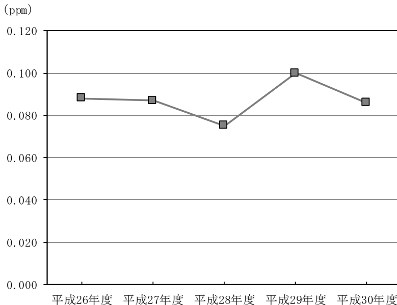
図 3.1-5 光化学オキシダントの昼間の 1 時間値の最高値の経年変化
