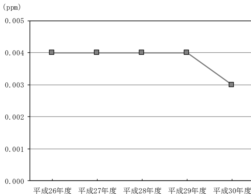
図3.1-4 二酸化窒素の年平均値の経年変化
