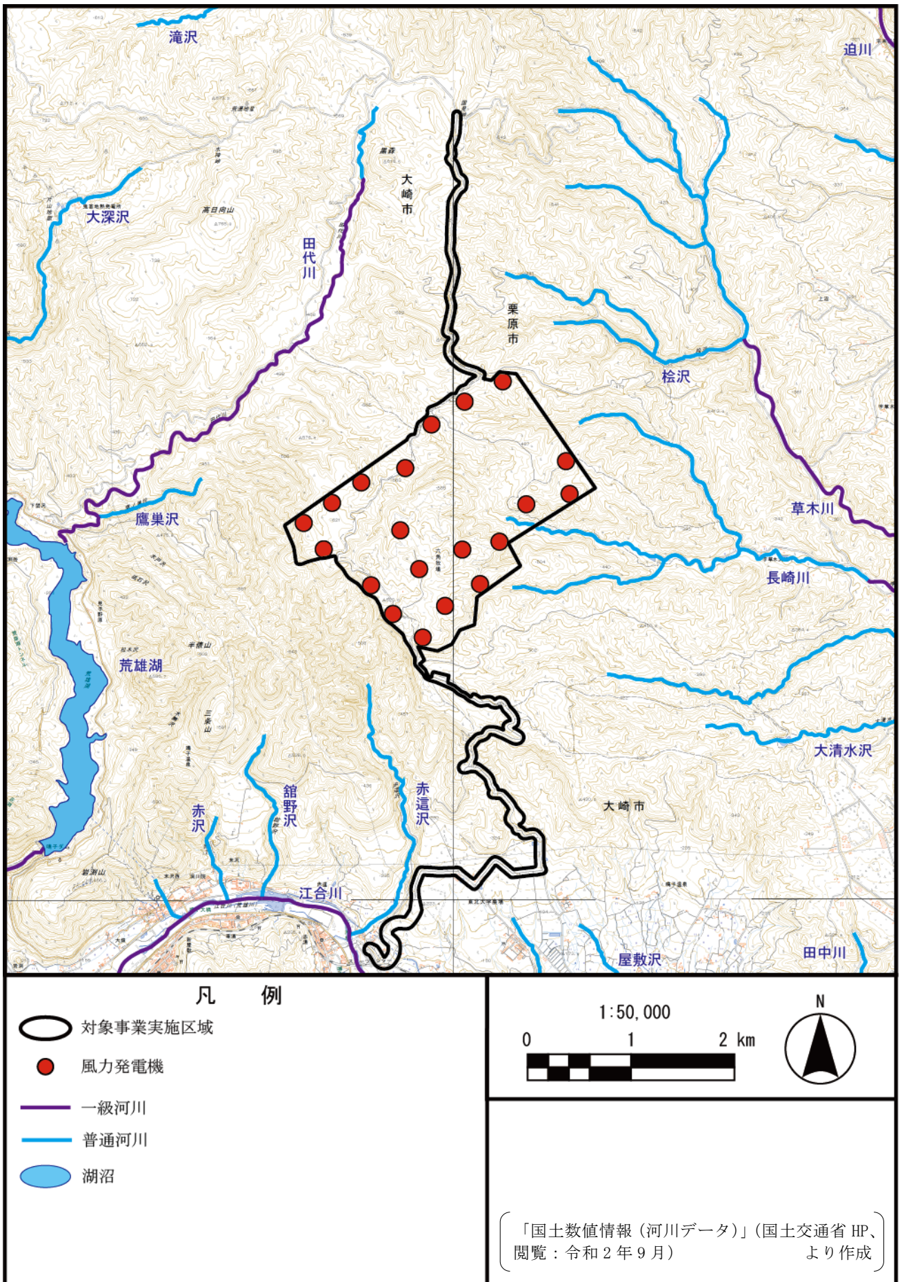
図 3.1-9 主要な河川及び湖沼の状況
