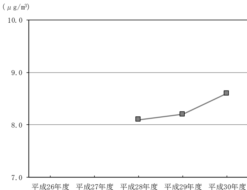
図 3.1-7 微小粒子状物質の年平均値の経年変化
