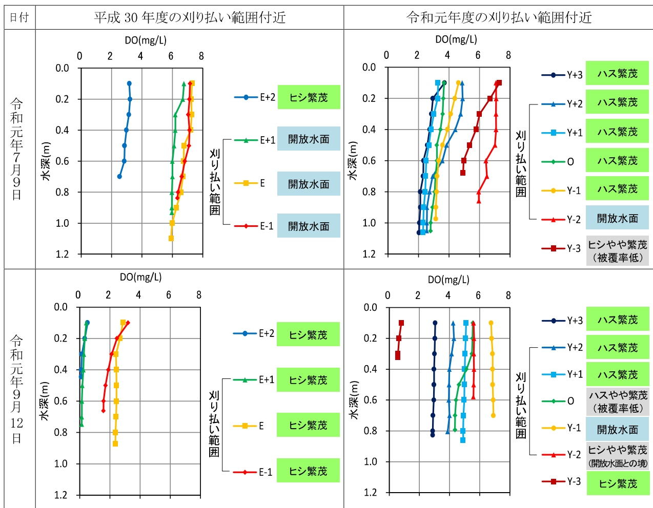
図 6 DO 鉛直分布
