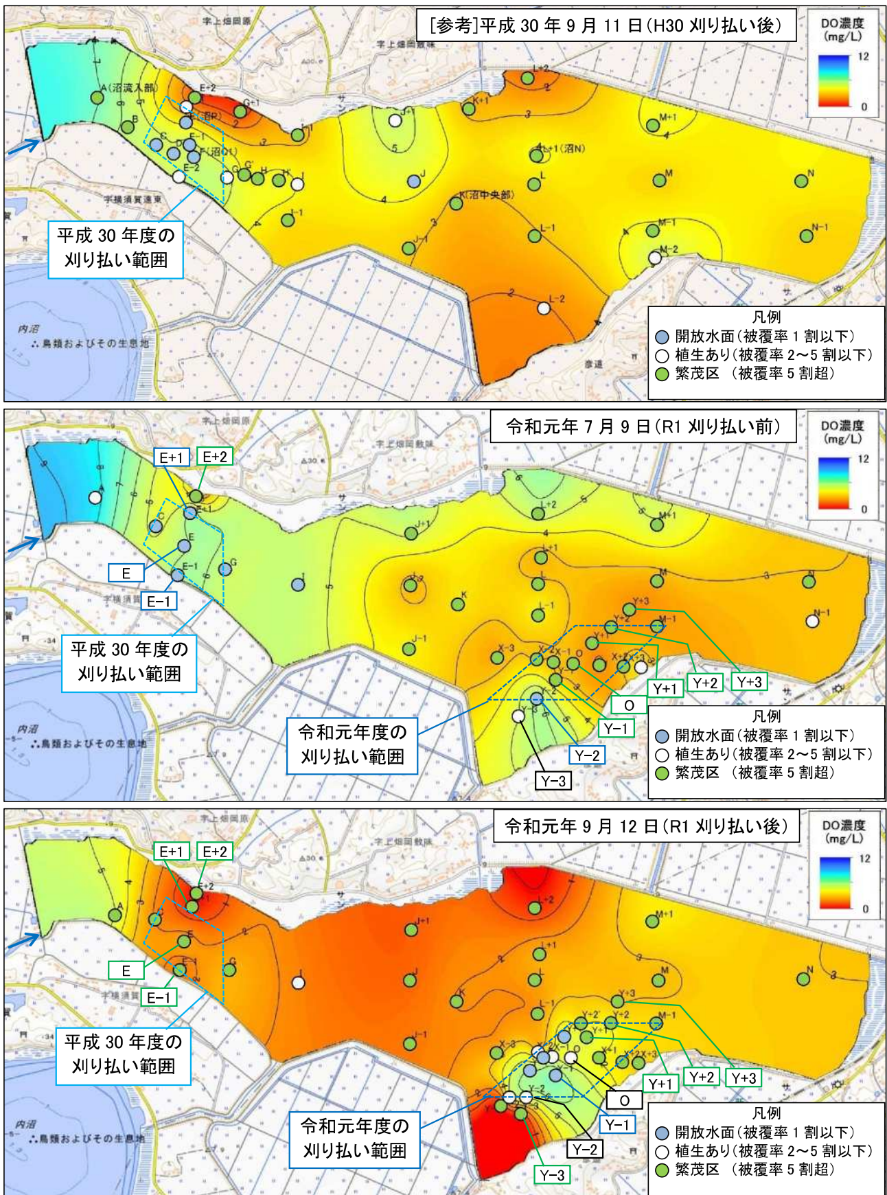
図 5 底層 DO 平面分布 (上段:H30/9/11、中段 : R1/7/9、下段 : R1/9/12)
