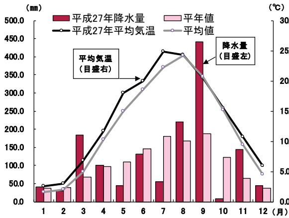
仙台市の月別平均気温と降水量
