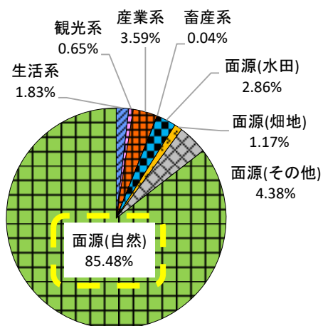
COD 排出負荷量の割合 (R3)
