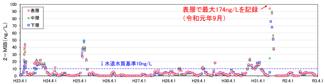
釜房ダム (ダムサイト) における 2-MIB 濃度の推移
