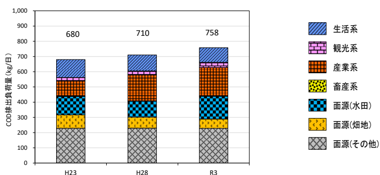
COD 排出負荷量のうち面源(自然) 2 を除いた経年変化
