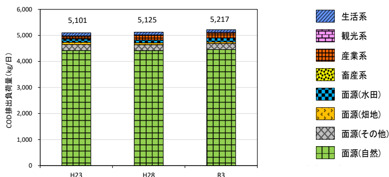
COD 排出負荷量の経年変化
