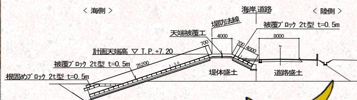
【標準断面図】
