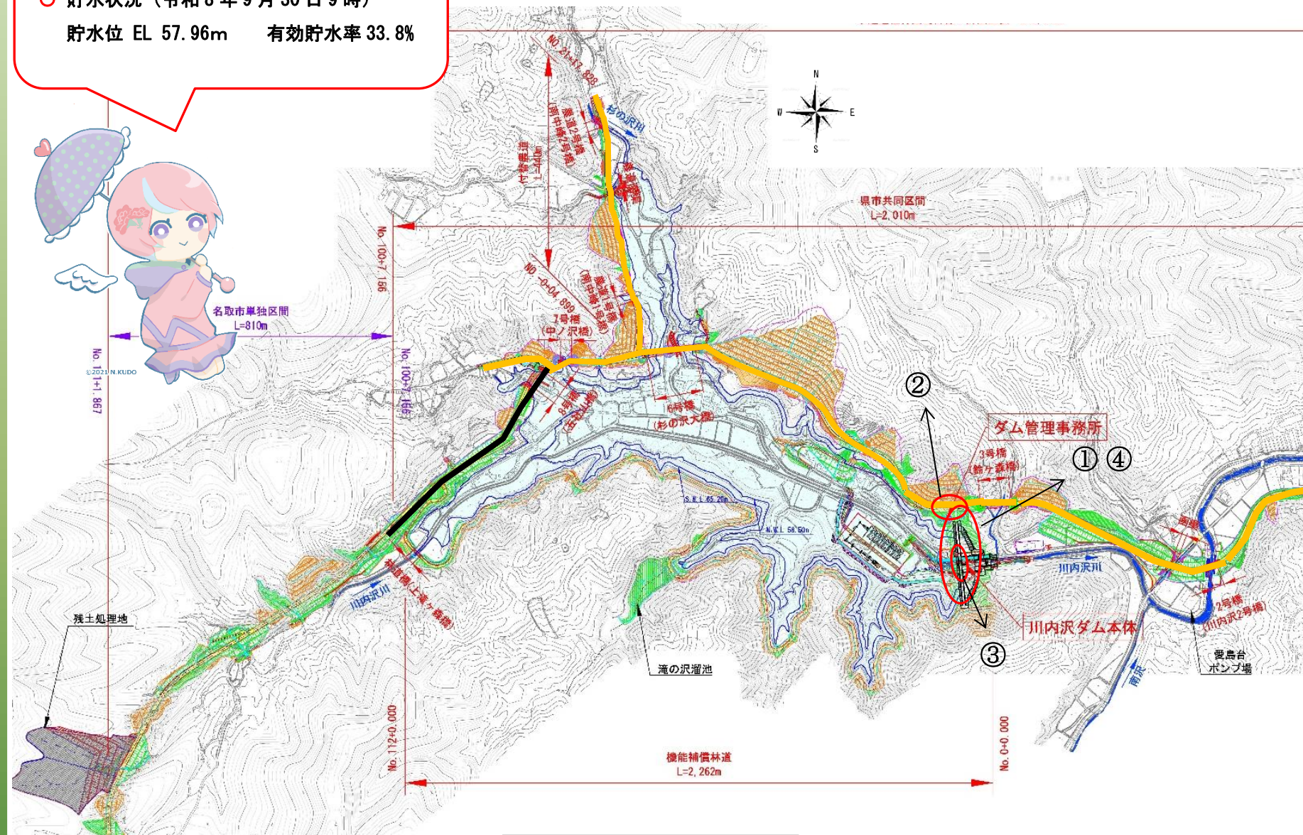
【③川内沢ダム管理設備工事】 右岸側 CCTV カメラ
