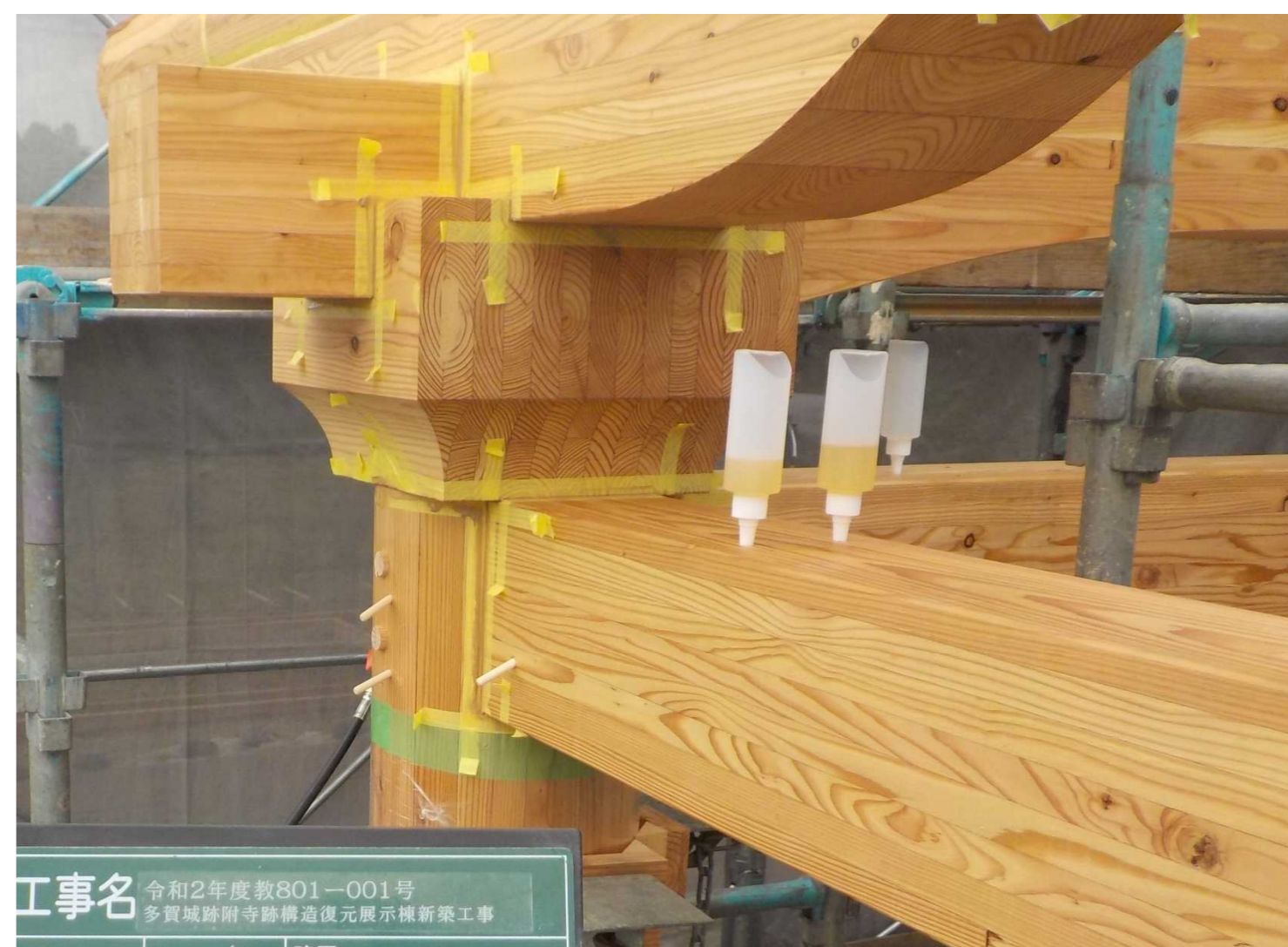
〔GIR工法施工状況〕
