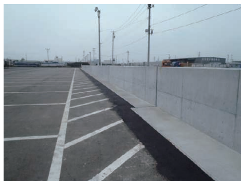
仙台港区防潮堤完成 (中野 6 号工区)
