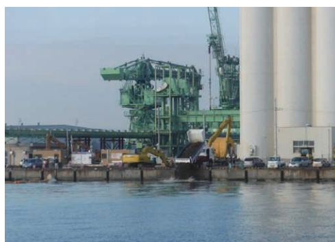
高松 2 号ふ頭埋立工事開始 (1.24)
