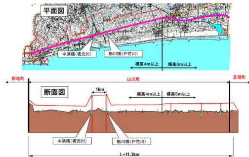
② 縦断計画
