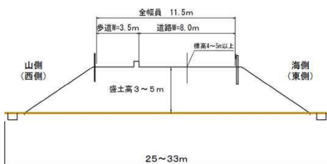
標準断面図(1/2)
