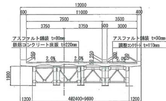
新設西川橋上部工断面図
