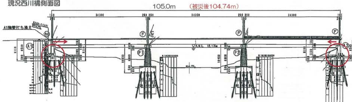
現況西川橋側面図
