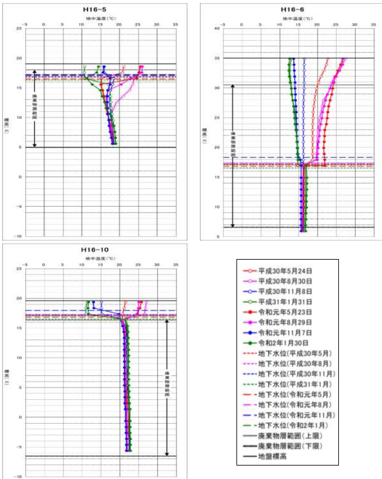
图 5-8 地中温度变化图 (浸透水) ②
