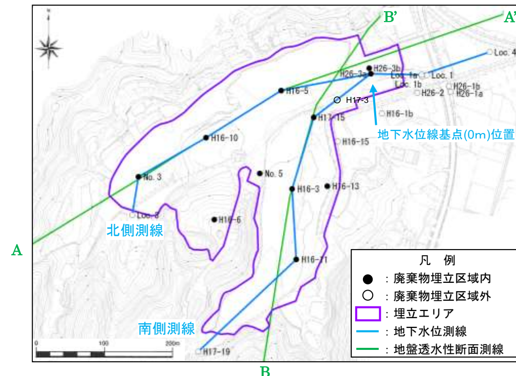
図5-14 令和元年度下半期の上流側～下流側にかけての水位標高変化（平面図）
