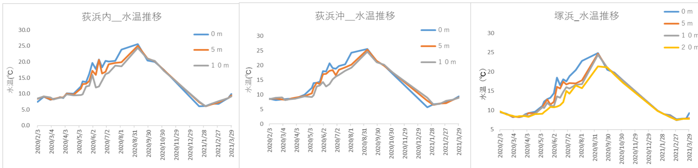
図 荻浜内湾、荻浜沖合、塚浜の水温の鉛直分布
