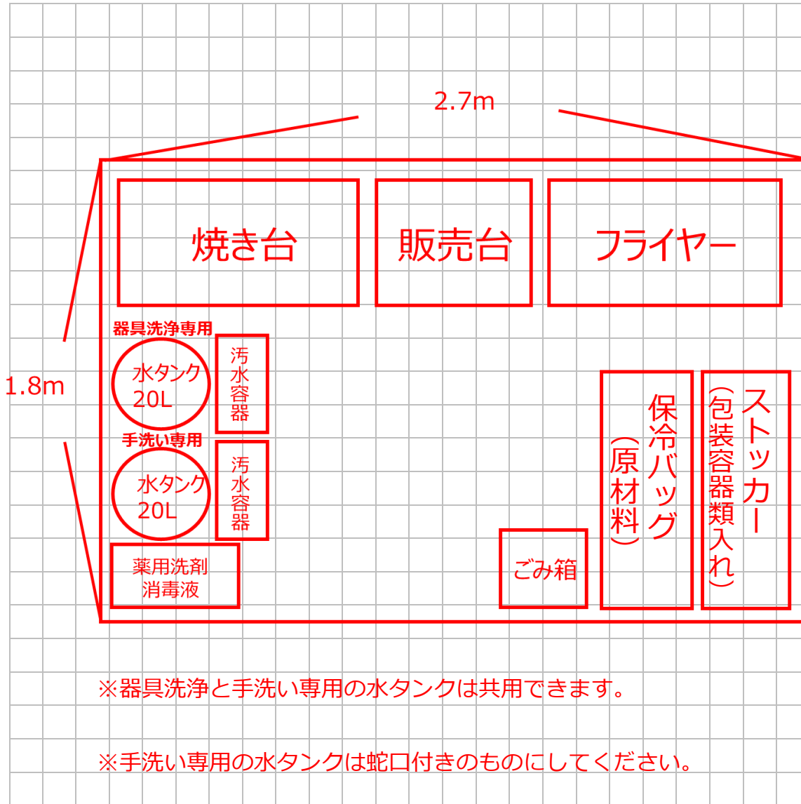
営業施設の平面図（一目盛 m）
