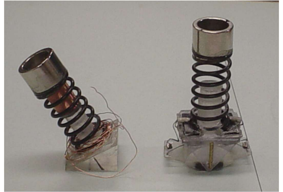
アクチュエータの概略
